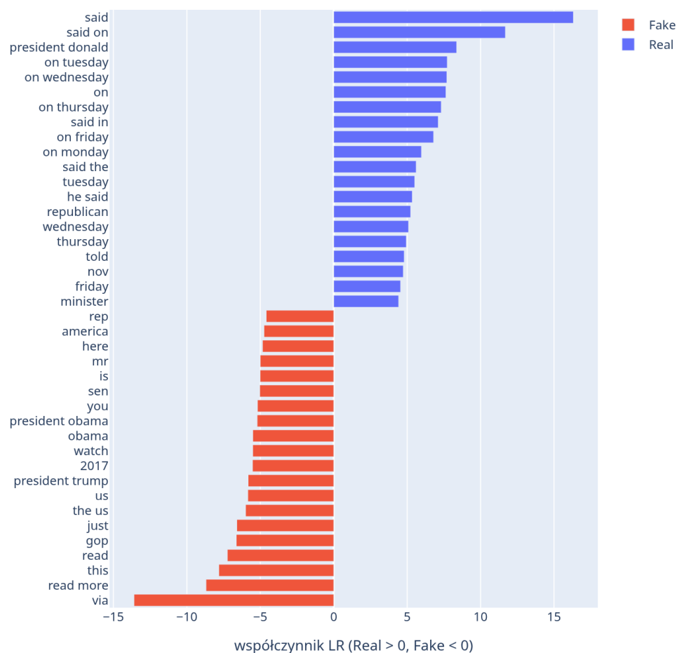
Rysunek 4: Najsilniejsze n-gramy wg współczynników regresji logistycznej ( \text{Real} > 0 , \text{Fake} < 0 ).
