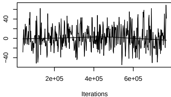
Trace of gwesp.OTP.fixed.0.5
