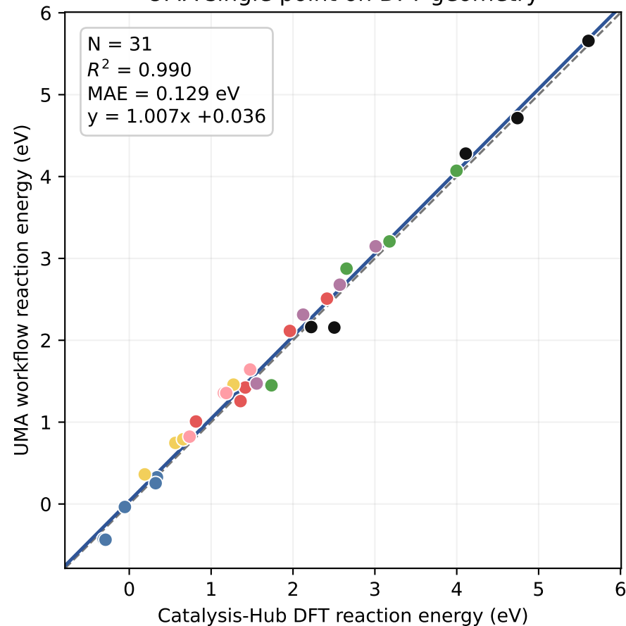
UMA single point on DFT geometry
