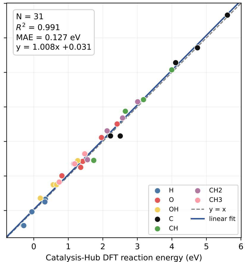
UMA constrained relaxation
