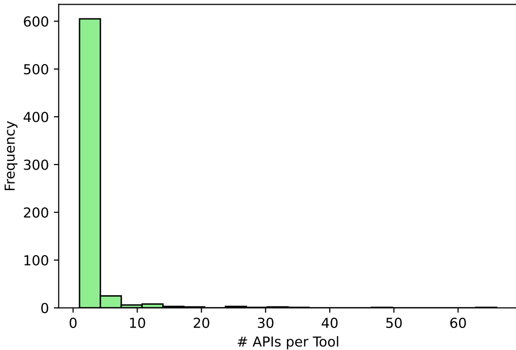
API Count per Tool
