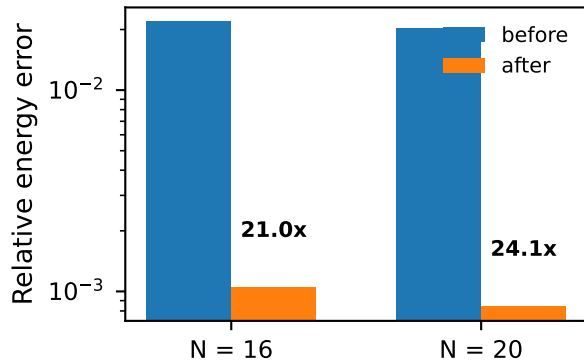
(d) J_2 / J_1 = 0.5 , exact
