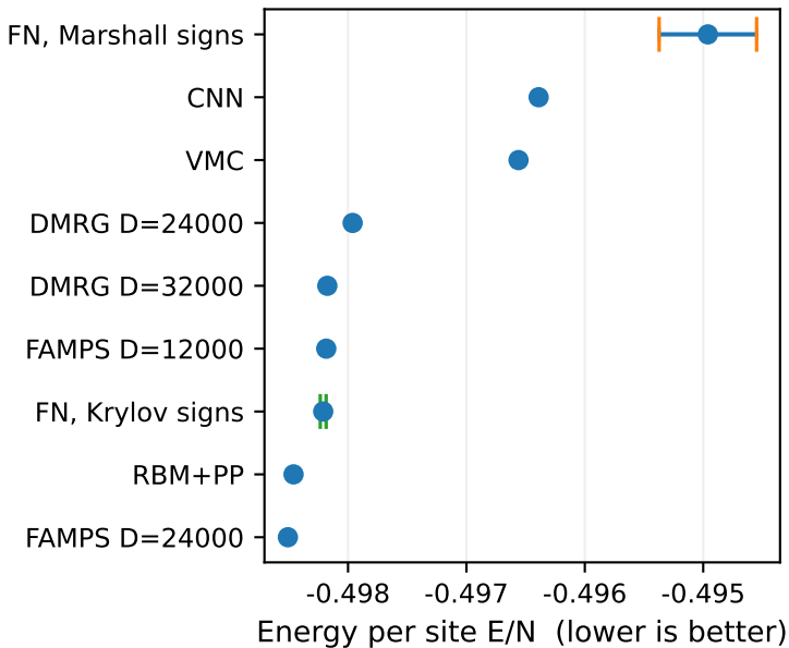
Periodic 8 x 8 lattice, J_2 / J_1 = 0.5
