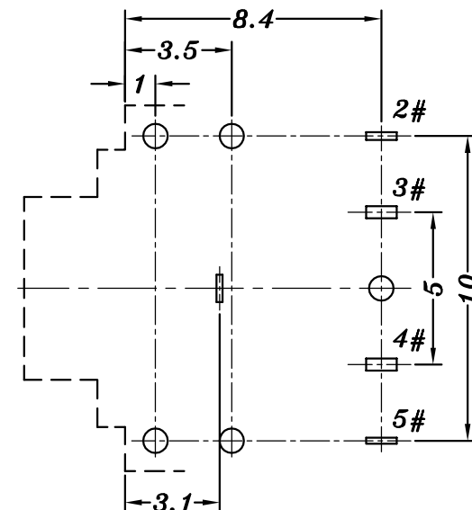
P.C.B LAYOUT
