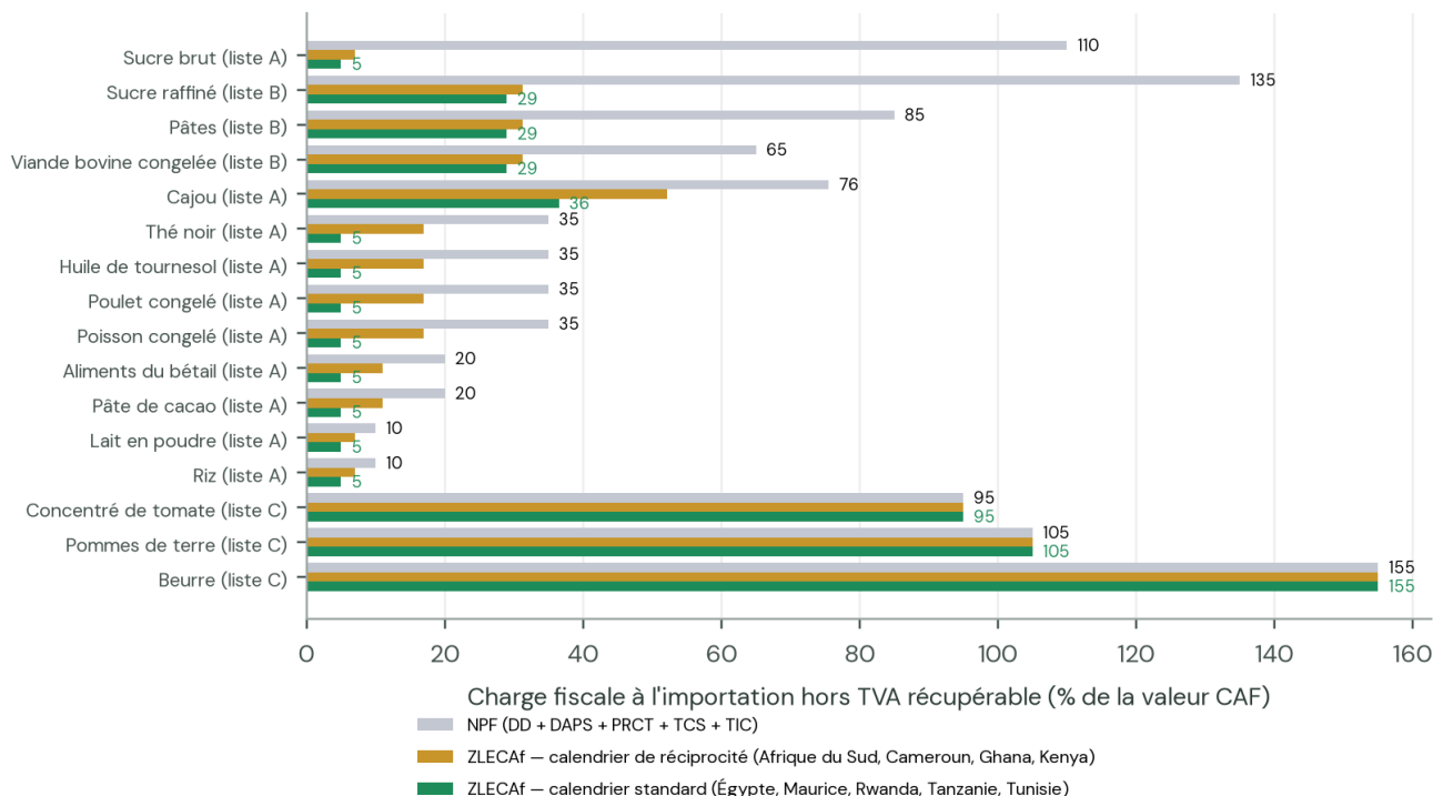
Figure 7.2 — Charge fiscale totale à l'importation en Algérie (hors TVA), NPF contre ZLECAF 2026
