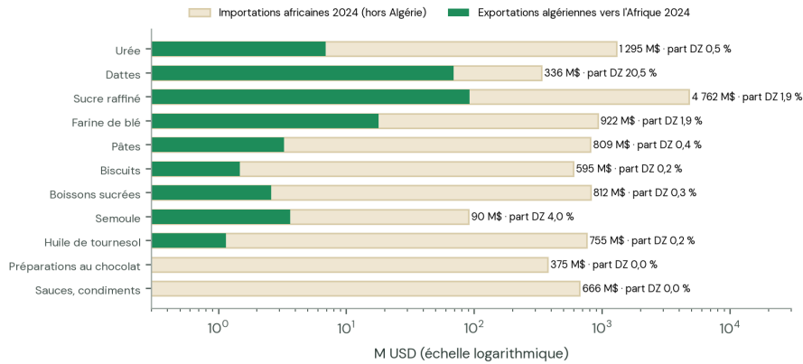
Figure 7.3 — Demande d'importation africaine 2024 et part captée par l'Algérie
