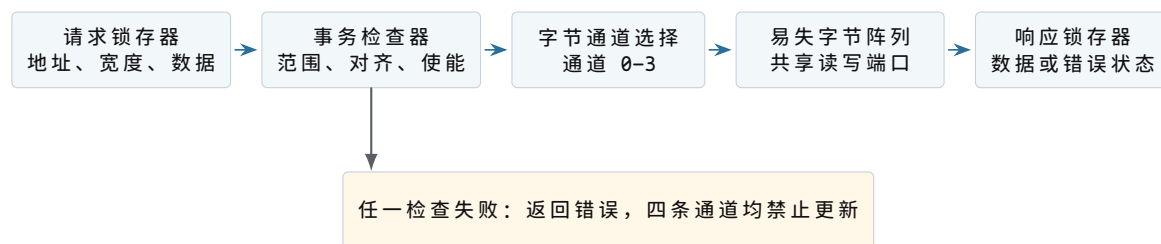
图示：写入的提交边界位于阵列端口；检查全部完成后，被使能字节在同一更新边界改变。响应锁存器中的 OK 表示这次阵列更新已经发生，而不是仅仅收到了写请求。
