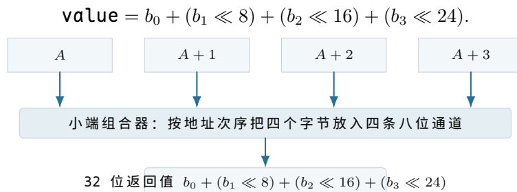
图示：字节顺序是处理器与存储接口之间的解释规则。RAM 单元只保存八个位，并不保存“最低有效字节”这个语义标签。
