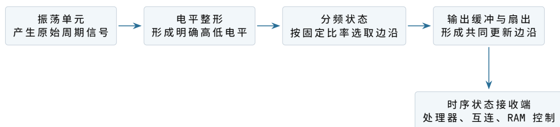
图示：分频状态和输出缓冲属于时钟路径本身；它们不构成软件可读计数器。处理器只能依赖状态在规定边沿更新，尚不能请求某个未来时刻的通知。
