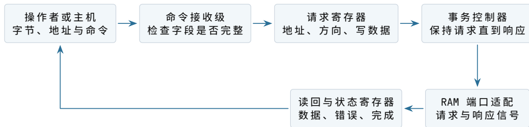
图示：夹具的提交边界是 RAM 响应到达并写入状态寄存器。主机发出命令并不等于 RAM 已经改变；读回核对也必须在对应事务完成以后进行。
