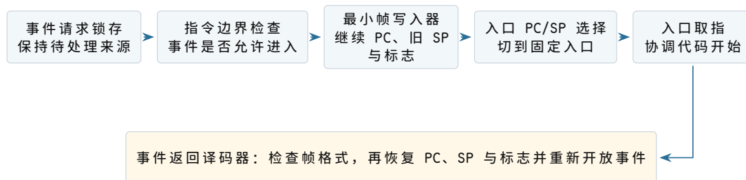
图示：异步入口不是把请求线直接接到 PC。处理器先等待精确指令边界，再建立可返回的最小帧，最后切换入口 PC/SP；事件返回只有在帧检查通过后才恢复被选中的执行流。
