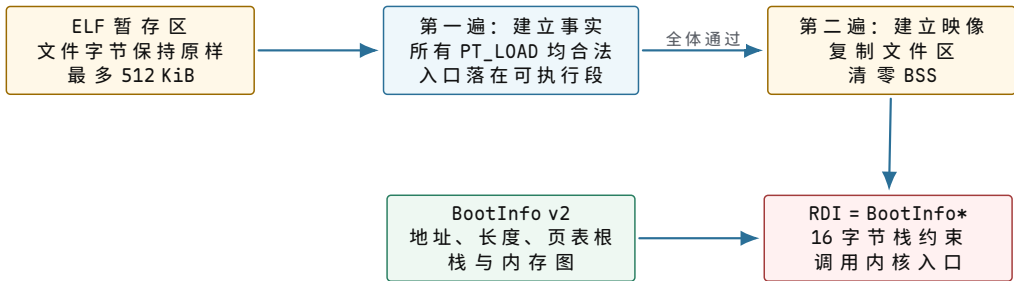
图示：ELF 校验、映像写入和 ABI 交接是三个边界。第一遍让失败仍可回滚，第二遍建立目标内存，BootInfo 再把启动事实交给内核。
