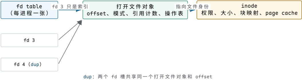
图示：整数 fd 只是进程 fd table 的索引；offset 和引用计数属于打开文件对象；inode 才是文件身份。dup 复制的是槽位，不是对象——这是后面所有共享 offset 现象的根源。
