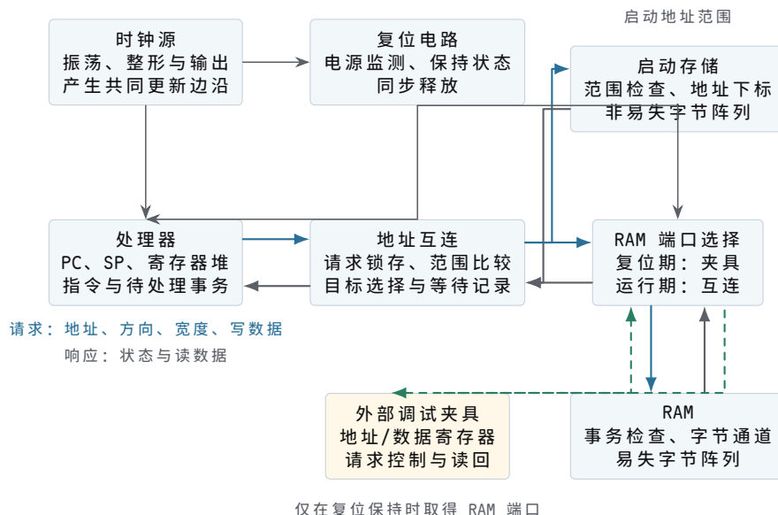
图示：蓝色箭头表示运行期请求，灰色箭头表示响应，虚线表示复位期间的人工准备通路。复位电路同时约束处理器与 RAM 端口选择器，因此调试夹具和处理器不会同时驱动 RAM。图中没有操作系统、调度器、系统调用或可编程计时器。
