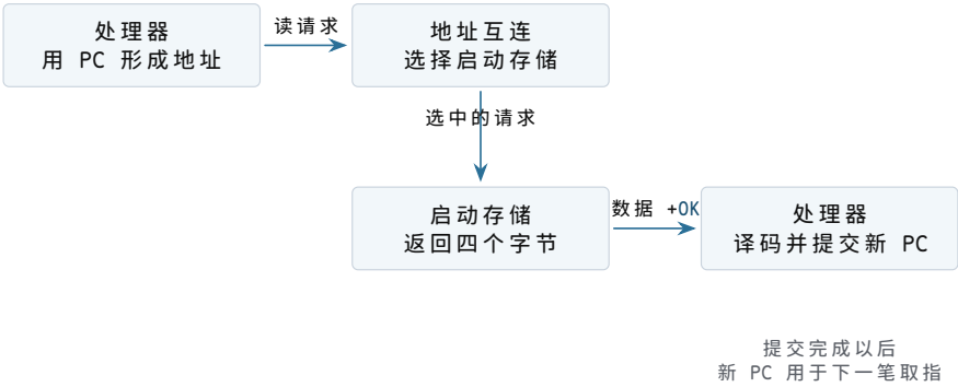
图示：取指不是处理器内部凭空取得指令。它是一笔带地址的读取事务；只有响应成功并完成译码后，处理器才提交新的 PC。
