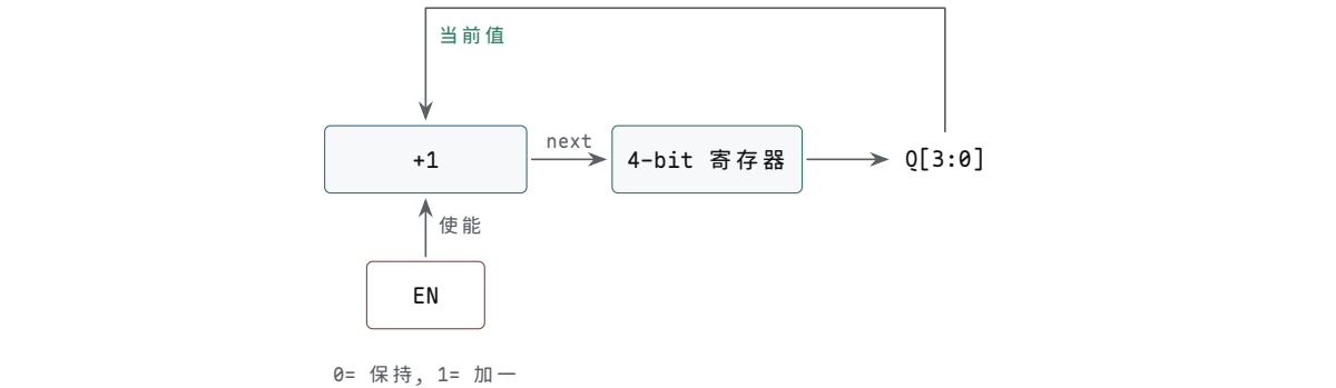
图示：4-bit 同步计数器。
