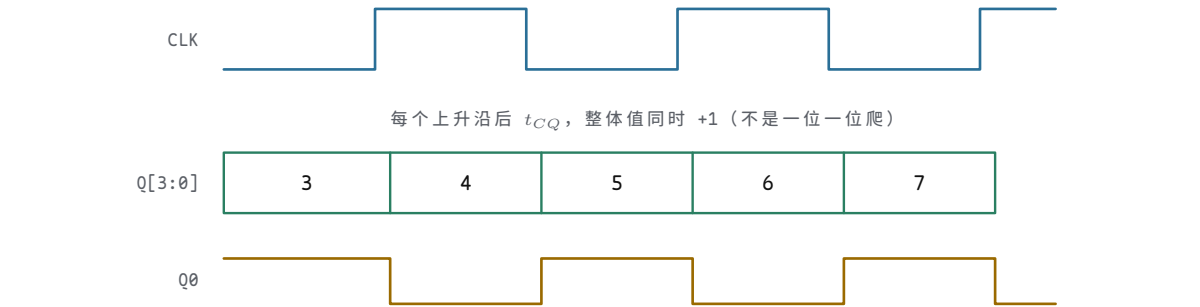
图示：4-bit 计数器波形：每个上升沿，寄存器把“当前值 +1”整体提交一次，总线带上的值从 3 整齐跳到 4、5、6、7。注意 Q0——它每个周期翻转，正好是 CLK 的二分频；Q1 再慢一半。计数器的每个 bit 都是比它低一位的半速时钟，这是后面分频和定时器的基础。
