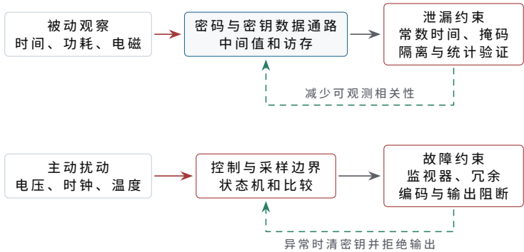
图示：侧信道与故障注入是两条相反的信息路径。侧信道从正常计算泄漏相关量，措施要降低“秘密-观测”的统计关系；故障注入从外部改变内部状态，措施要在结果发布前检测异常并阻断输出。两类措施不能互相替代。
