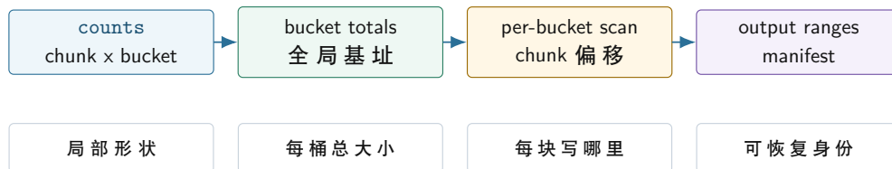
多路 partition 的二维前缀
