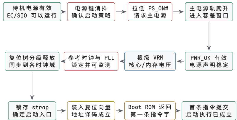
图示：ATX 类平台的一次冷启动放行链。待机域先处理按键和策略，PS_ON# 只请求主电源开始工作；主电源、板级 VRM、参考时钟和各级复位依次建立条件。复位释放之后还要成功锁存启动配置、命中复位向量、从不可变入口取得合法指令并完成首条提交，才能说处理器真正开始执行。
