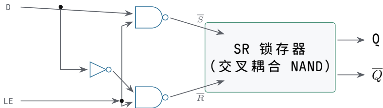
图示：D 锁存器的门级实现：LE=1 时，D 和它的反相信号分别推开两扇 NAND，一路 \overline{S} 或 \overline{R} 被拉低（写入）；LE=0 时两扇都关闭， \overline{S} 、 \overline{R} 同为高（保持）。0,0 禁行从结构上不可能再出现——这就是“把 set/reset 两条危险命令合并成 D 和 LE”在电路结构上的直接体现。
