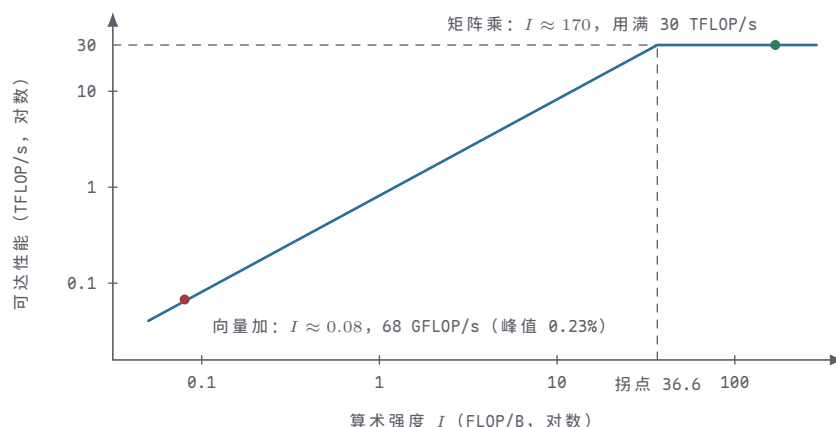
图示：双对数坐标下的 roofline：斜段是带宽屋顶（可达性能 = 带宽 × 算术强度），平段是算力屋顶 30 TFLOP/s，拐点 I^* = 30000/820 \approx 36.6 FLOP/B。向量加的强度只有约 0.08 FLOP/B，被带宽屋顶压在 68 GFLOP/s—峰值的 0.23%；矩阵乘约 170 FLOP/B，远在拐点右侧，峰值真正用满。横轴每往左一格，同样的算力折扣再重一倍。
