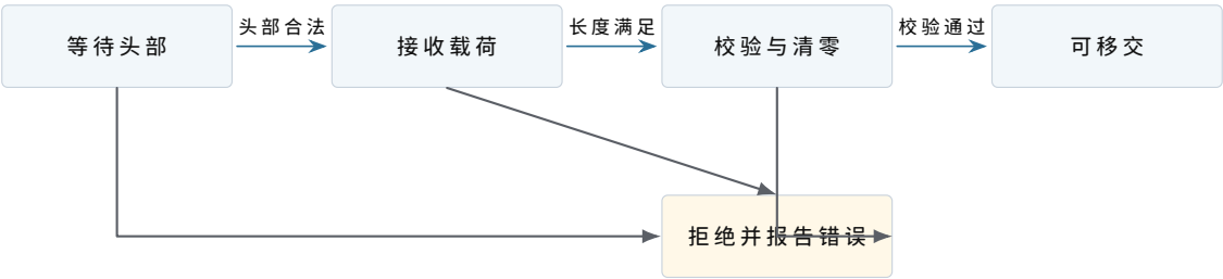
图示：“载荷到齐”只关闭接收阶段；只有校验、零填充和布局建立全部成功，装入记录才进入“可移交”。任何失败都不能改变 PC 到任务入口。
