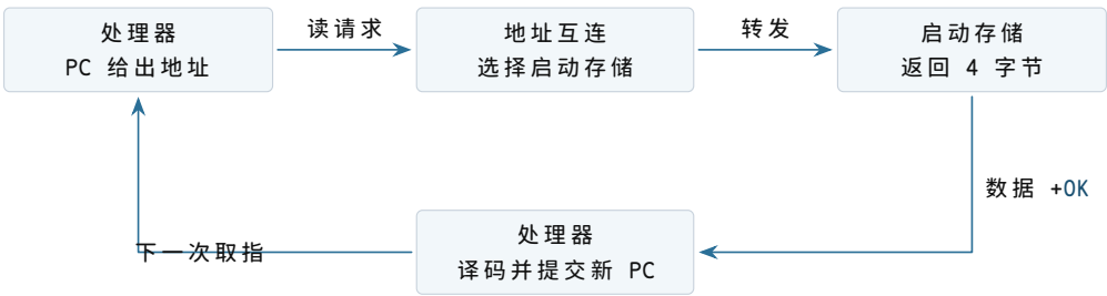
图示：取指不是处理器内部凭空取得指令。它是一笔带地址的读取事务；只有响应成功并完成译码后，处理器才提交新的 PC。
