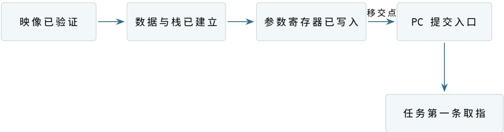
图示：“字节已经在 RAM 中”和“任务已经运行”之间隔着初始现场建立与 PC 提交。只有最右侧事件改变取指来源。
