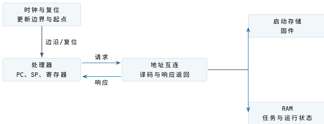
图示：此时机器已经能从固定固件取指并访问 RAM，但 RAM 中尚无可靠任务字节。地址互连只负责送达，不负责决定“今天运行哪个任务”。
