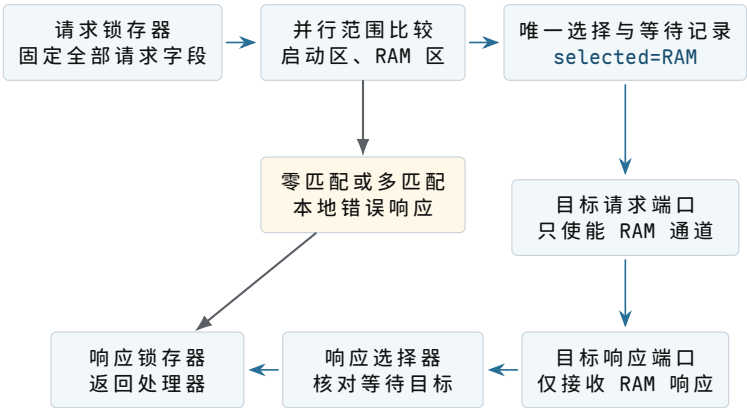
图示：地址 0x00102004 使 RAM 比较结果为 1。互连把这一位选择和请求字段一起保持到响应返回，因此较晚到达的响应仍能被送回正确事务；零匹配或多匹配由互连直接报错。
