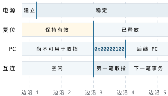
图示：电源稳定并不立即开始取指。复位先保持若干边沿，释放后才把规定的 PC 值用于第一笔事务；第一条指令完成后，PC 才进入后继值。
