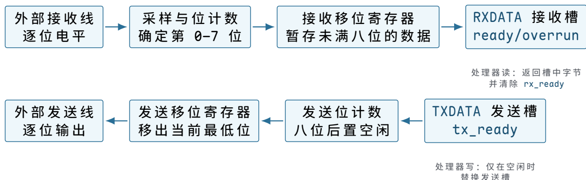
图示：上排把外部位流提交为一个软件可读字节，下排把一个软件提交的字节展开成位流。接收槽和发送槽是两个独立所有权边界，不能用一根“串口缓冲”线概括。
