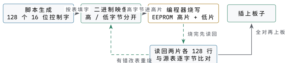
图示：微码 ROM 的烧写流程。脚本按微操作表生成 128 个 16 位控制字，高字节烧进高片、低字节烧进低片；烧完先用编程器把两片各 128 行读回，与源表逐字节比对，全对再上板。跳过读回直接上板，会把烧写错误混进接线错误里一起排查——两类故障症状一样，区分它们只需要一次读回。
