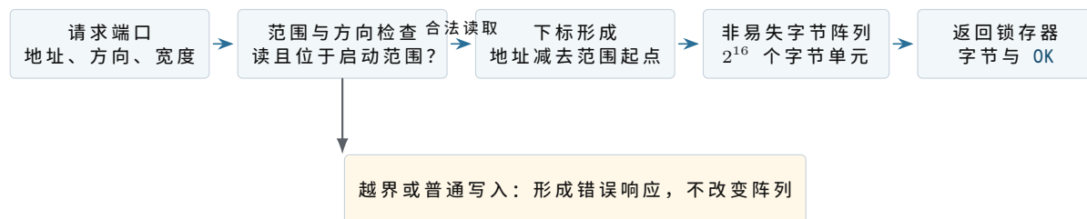
图示：启动存储内部真正保存的是非易失字节阵列。检查器、下标形成和响应锁存器负责把外部事务变成一次稳定读取；它们不为字节附加“指令”或“固件”标签。
