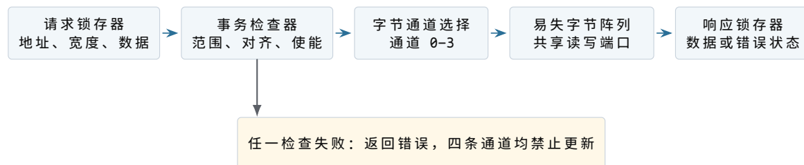
图示：写入的提交边界位于阵列端口；检查全部完成后，被使能字节在同一更新边界改变。响应锁存器中的 OK 表示这次阵列更新已经发生，而不是仅仅收到了写请求。
