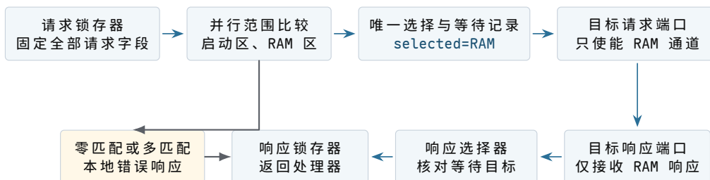
图示：地址 0x00102004 使 RAM 比较结果为 1。互连把这一位选择和请求字段一起保持到响应返回，因此较晚到达的响应仍能被送回正确事务；零匹配或多匹配由互连直接报错。
