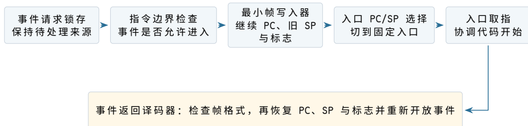
图示：异步入口不是把请求线直接接到 PC。处理器先等待精确指令边界，再建立可返回的最小帧，最后切换入口 PC/SP；事件返回只有在帧检查通过后才恢复被选中的执行流。
