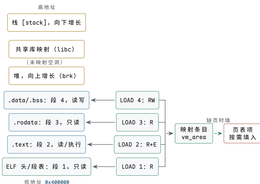
图示：进程地址空间从低地址到高地址的布局（对应正文 hello 例）：主程序四个 LOAD 段从 0x400000 起依次排开，堆紧随其后向上增长，共享库映在 0x7f... 区间，栈在最高处向下增长，各区之间隔着未映射的空洞。右侧是
