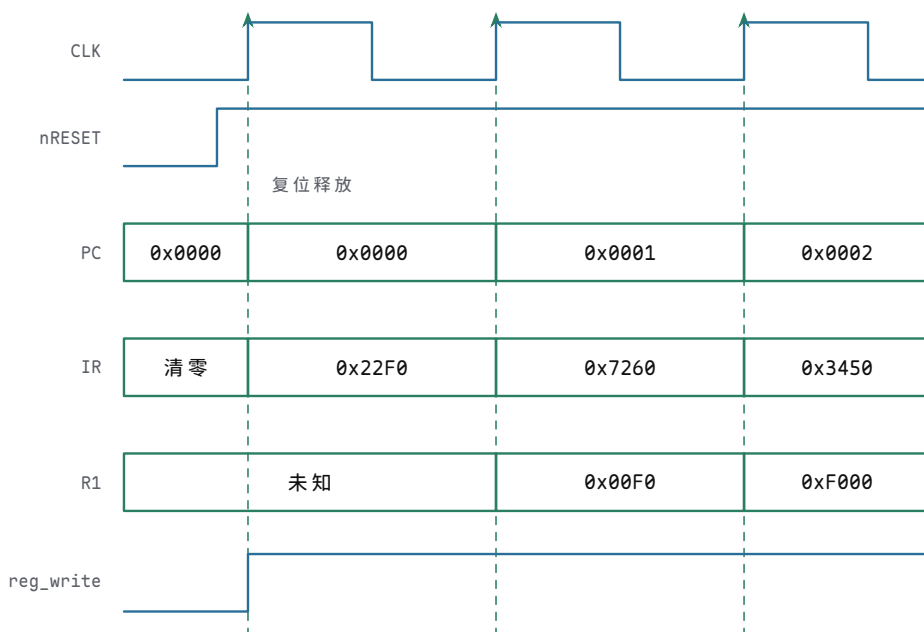
图示：复位后前三个周期的时序，对照“极小 ISA 与可接线数据通路”一节 ROM 程序开头三条编码（ 0x22F0=MOV\ R1, 0xF0 、 0x7260=SHL\ R1, 8 、 0x3450=MOV\ R2, [R1+4] ）。复位把 PC 保持在 0x0000 、写使能保持在安全值；释放后每个周期内组合路径完成取指、译码、执行，周期末上升沿才提交新状态— 0x00F0 在第二个上升沿、 0xF000 在第三个上升沿写进 R1。这张波形图直观展示了“状态只在时钟沿改变”，单步调试时应逐格核对。
