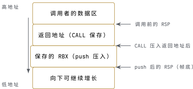
图示：函数调用案例对应的栈帧内存布局。CALL 先把返回地址压入，RSP 下移一格； sum2 的序言用 push 把 RBX 保存到新帧里；尾声 pop 按相反顺序恢复，RSP 加回。RET 硬件只认“返回地址”这一格：若某条越界写改写了它，RET 就把被污染的值装进 PC，程序表现为“返回后失控”。
