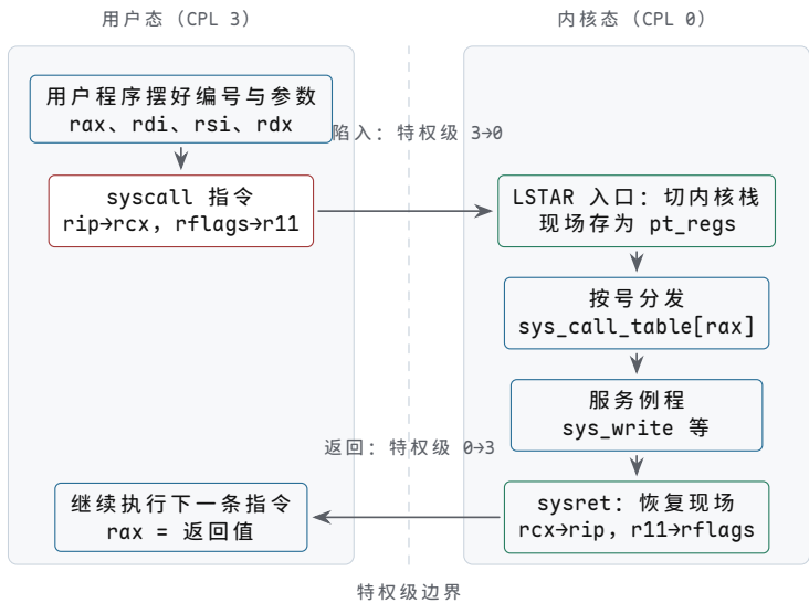
图示：一次系统调用往返的泳道图：左为用户态（CPL 3），右为内核态（CPL 0），中间虚线是特权级边界，两次越界即 CPL 3→0 与 0→3 的切换点。syscall 指令把返回地址与标志装进 rcx/r11、把 rip 换成 MSR 中的内核入口；入口代码切到本进程内核栈，把全部通用寄存器存成 pt_regs，再按 rax 中的编号查 sys_call_table 分发；服务完成后 sysret 逆向恢复。内核全程不必解引用用户栈指针。
