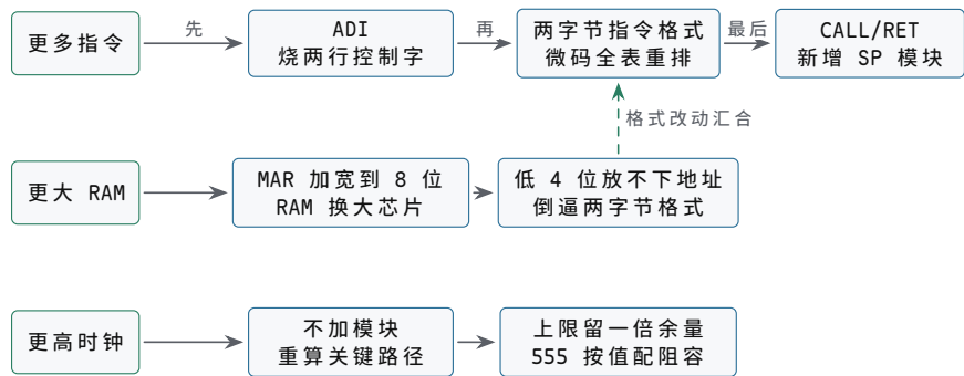
图示：扩展路径决策（对应正文扩展方向表）。三个目标各有走法：加指令按成本递增排——ADI 只烧两行控制字，最便宜；两字节指令格式要重排全表微码；CALL/RET 与栈要新增 SP 计数器模块，最贵。扩 RAM 连锁最多：MAR 加宽、RAM 换大之外，低 4 位放不下地址，同样倒逼两字节格式。提高时钟不加模块，只重算“总线到 ALU 到 A 建立时间”这条关键路径，理论上限再留一倍余量。所以扩展的顺序不是随机的：先有栈才谈得上子程序，再有富余的地址空间才谈得上中断向量。
