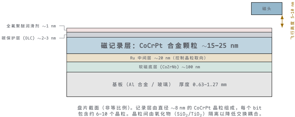
图示：盘片多层薄膜结构。实际各层厚度比图中比例小得多——记录层仅 15–25 nm，碳保护层仅 2–3 nm。基板表面粗糙度 <0.3\text{ nm Ra} 。
