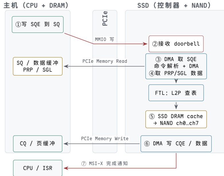
图示：NVMe 命令处理流程。64K 队列 \times 64K 深度允许数万条命令同时在途 (in-flight)，远超 AHCI 的单队列 32 深度。多队列可绑定到不同 CPU 核，消除锁竞争。
