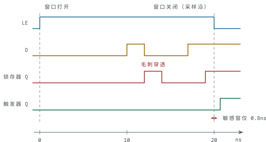
图示：同一个 D 送到两种元件：LE 窗口 ( t=0 到 20ns) 内， D 上 2ns 宽的毛刺 ( t=10 ns) 和晚到的变化 ( t=17 ns) 都经过约 2ns 延迟穿透到锁存器 Q ； D 触发器只认 t=20 ns 采样沿前后共 0.8ns 的窗口，毛刺完全不可见，晚到变化被正常采入，沿后 Q 一步更新。敏感区 20ns 对 0.8ns，相差 25 倍——这就是透明窗口的代价。
