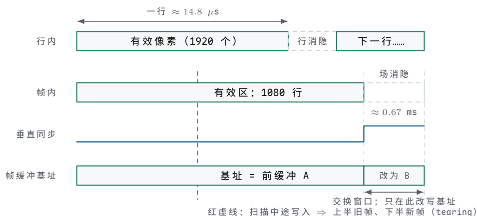
图示：显示扫描的两层时序（示意，不按比例）：行内先发有效像素再入行消隐，一行约 14.8 \mu\text{s} ；帧内扫完 1080 个有效行入场消隐，垂直同步脉冲随之拉高。双缓冲的交换——改写帧缓冲基址寄存器——只允许发生在职消隐窗口内；若在扫描中途改写（红虚线），屏幕上半是旧帧、下半是新帧，这就是 tearing。
