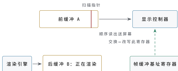
交换只在职消隐那 0.67 \text{ ms} 内执行：一次寄存器写，零拷贝，A、B 角色互换
