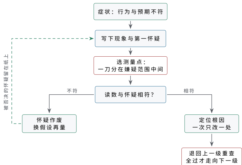
图示：故障排查决策树（对应联调日志六步的走法）。症状写下后提出第一怀疑，怀疑的职责是指定第一个测量点——选在与各嫌疑都无关、一刀分在范围中间的位置量；读数与怀疑不符，怀疑就地作废、换假设再量；相符才动手，一次只改一处；改完退回上一级重查，本级全过才允许走向下一级。日志里六个坑平均八十分钟一个，靠的就是这条看起来慢的纪律。
