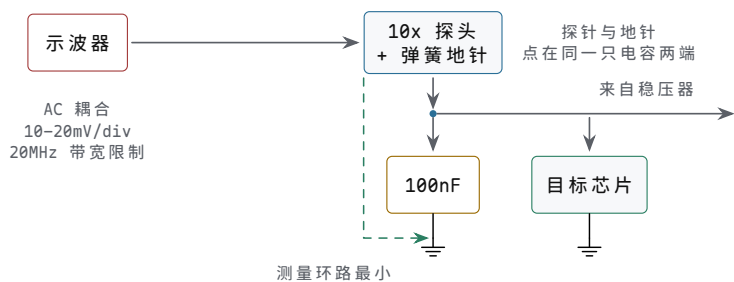
图示：纹波测量的标准接法。示波器切 AC 耦合挡住直流分量，用 10-20mV/div 的档位把纹波展开；10x 探头配弹簧地针，探针与地针直接点在同一只电容的两端——测的是负载端真实看到的电源，探头围出的测量环路也最小；示波器若有 20MHz 带宽限制就打开，挡住与电源无关的高频拾取。
