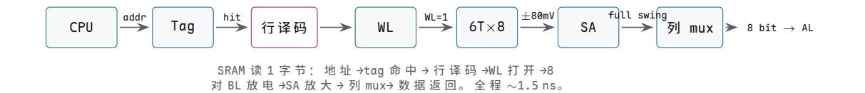
图示：SRAM 读路径。每一步都是组合逻辑或单级放大，没有等待状态，因此 L1 访问可以在一个时钟周期内完成。
