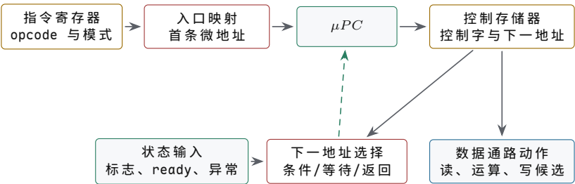
图示：微序列器的闭环。主指令通过入口映射给出首条微地址；控制存储器同时输出数据通路控制和下一地址信息；标志、ready 与异常参与下一地址选择。只有结束微指令到达提交条件后，主指令才完成， \mu PC 的中间推进不是架构完成。
