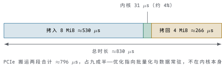
图示：一次内核启动的耗时构成 ( N = 2^{20} 向量加, PCIe 3.0 x16, 按比例)：拷贝 8 MiB 约 530 \mu s, 内核执行约 31 \mu s, 拷回 4 MiB 约 266 \mu s, 总时长约 830 \mu s。两次 PCIe 搬运占九成半, 内核只占约 4%—算术强度约 0.08 FLOP/B 的负载, 时间几乎全花在搬运上；工程上要么批量化、让数据常驻显存把这笔固定开销摊薄, 要么干脆留在 CPU 上。
