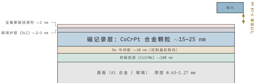
盘片截面（非等比例）。记录层由直径 \sim 8\text{ nm} 的 CoCrPt 晶粒组成，每个 bit 包含约 6–10 个晶粒。晶粒间由氧化物（ \text{SiO}_2/\text{TiO}_2 ）隔离以降低交换耦合。
