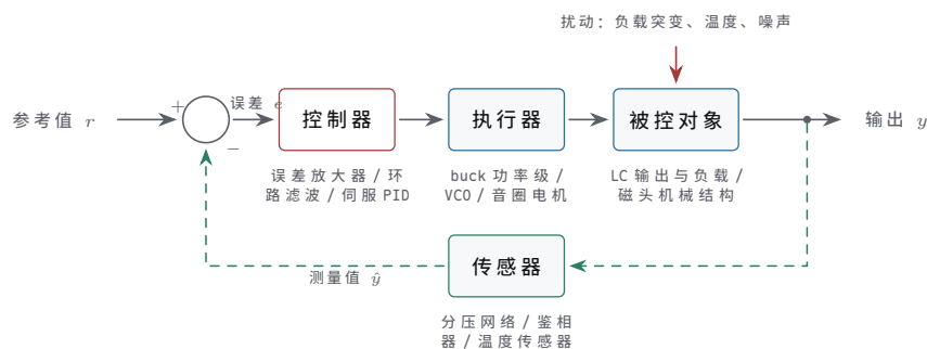
图示：通用反馈环。实线是前向通路：参考值与测量值在求和点相减得到误差，控制器按误差计算控制量，经执行器作用于被控对象；虚线是反馈通路：传感器测量输出并送回求和点。扰动从前向通路中途进入——这是反馈存在的理由：
