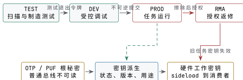
图示：生命周期与密钥路径必须互相约束。PROD 状态参与派生，返修前先清除任务数据并使旧工作密钥不可再生；否则“重新打开调试”会同时重新打开任务期秘密。状态转换、密钥版本和调试能力属于同一次不可逆提交。
