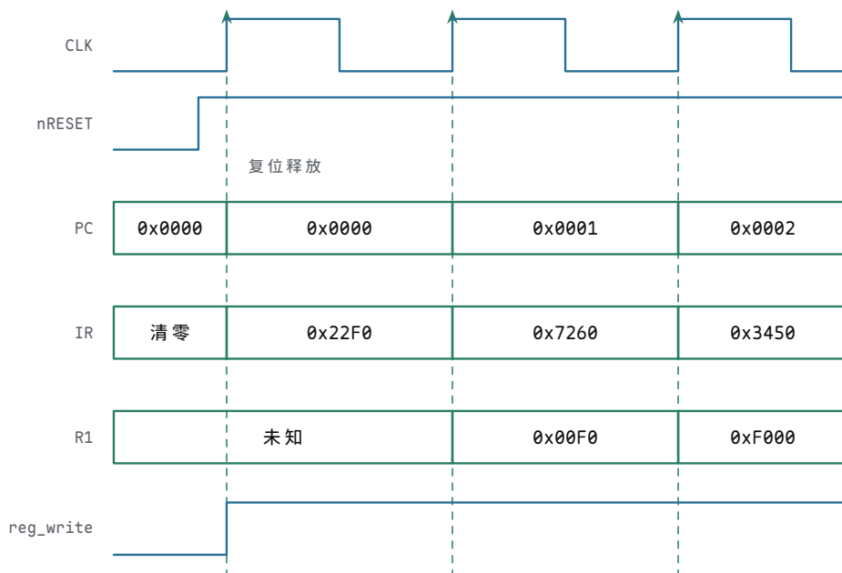
图示：复位后前三个周期的时序，对照“极小 ISA 与可接线数据通路”一节 ROM 程序开头三条编码（ 0x22F0=MOV R1, 0xF0 、 0x7260=SHL R1, 8 、 0x3450=MOV R2, [R1+4] ）。复位把 PC 保持在 0x0000 、写使能保持在安全值；释放后每个周期内组合路径完成取指、译码、执行，周期末上升沿才提交新状态—— 0x00F0 在第二个上升沿、 0xF000 在第三个上升沿写进 R1。这张波形图直观展示了“状态只在时钟沿改变”，单步调试时应逐格核对。
