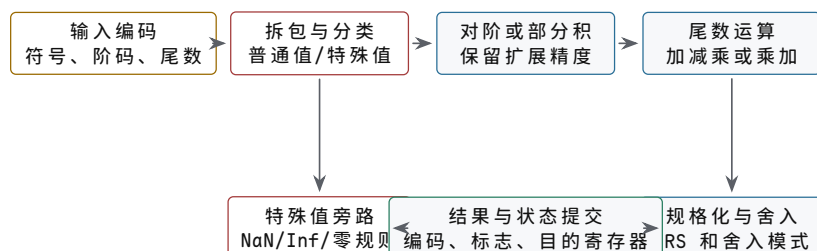
图示：浮点流水先分类，再分成普通数值路径和特殊值旁路。普通路径保留比目标格式更多的内部位，直到规格化完成后才按当前模式舍入；特殊值路径独立判定 NaN、无穷大和零的结果。两条路径在结果编码与异常状态的共同提交点汇合。
