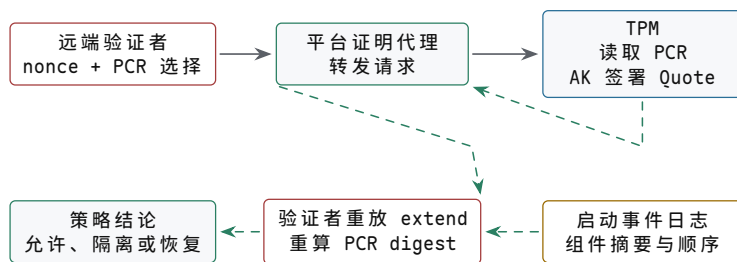
图示：远程证明的两类证据。Quote 由 TPM 签名，保护 PCR 摘要和本次 nonce；事件日志通常位于普通内存或固件存储中，本身可以被篡改，但篡改后的重放结果无法与签名保护的 PCR digest 对上。验证完成的可见结果是策略结论，不是 TPM 自动把机器判为“安全”。
