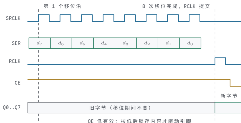
图示: 74HC595 串并转换时序 (括号内为部分手册别名: SER=DS、SRCLK=SHCP、RCLK=STCP); SRCLK 的 8 个有效沿把 SER 上的 d_7 到 d_0 逐位移入内部移位寄存器, 期间输出锁存器保持旧字节, 外部引脚纹丝不动; 8 次移位完成后给一个 RCLK 沿, 整字节一次性提交到 Q0..Q7; OE 低有效, 拉低之前引脚呈高阻。内部状态推进与外部可见提交分开, 正是这颗芯片输出不抖的原因。
