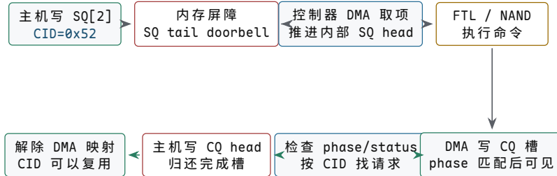
图示：一条 NVMe 命令的两次所有权交接。上排由主机发布 SQ 槽，doorbell 只扩大控制器可取范围；下排由控制器发布 CQ 槽，主机只有在 phase 匹配且 status 合法后才消费。CID 解决“完成属于哪笔命令”，phase 解决“这个数组槽属于哪一圈”，generation 还要解决“完成属于复位前还是复位后”。
