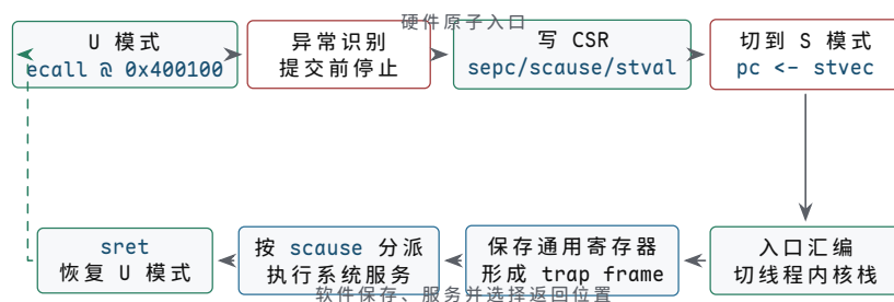
图示：一次 U 模式 ecall 的完整交接。上行由硬件在提交边界原子完成：记录故障 PC 与原因、保存先前特权状态、切换模式并装入向量入口；下行由入口汇编和内核完成：切栈、保存通用状态、分派服务，最后由 sret 恢复先前模式。硬件没有自动切到线程内核栈，因此“已进入 S 模式”和“已经有安全的内核栈”是两个不同边界。
