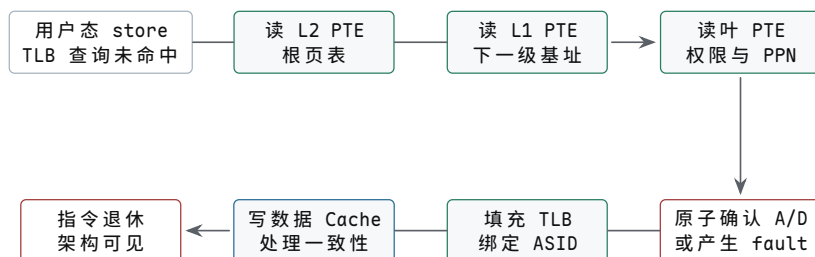
图示: TLB miss 只选择硬件页表遍历路径, 不等于 page fault。遍历必须取得合法叶项, 完成必要的 A/D 位更新, 填充带 ASID 的翻译, 再把数据写入 Cache; 只有 store 到达处理器规定的退休边界, 软件才观察到该指令完成。
