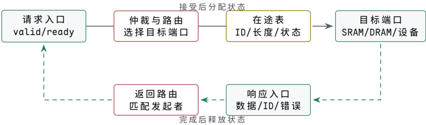
图示：多笔在途事务的状态闭环。请求在握手沿被接受后占用一项在途状态；响应按 ID 返回并累计 beat，只有数据完整或错误被确认后才会释放。请求、接受、响应与完成是四个不同边界。
