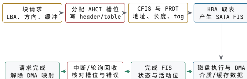
图示：AHCI/SATA 的所有权闭环。上排由驱动建立命令槽、CFIS 和 PRDT，发布后 HBA 才能取表并在链路上发出 FIS；下排由设备传输数据并返回完成状态，驱动核对槽位后才结束请求、解除 DMA 映射并复用内存。
