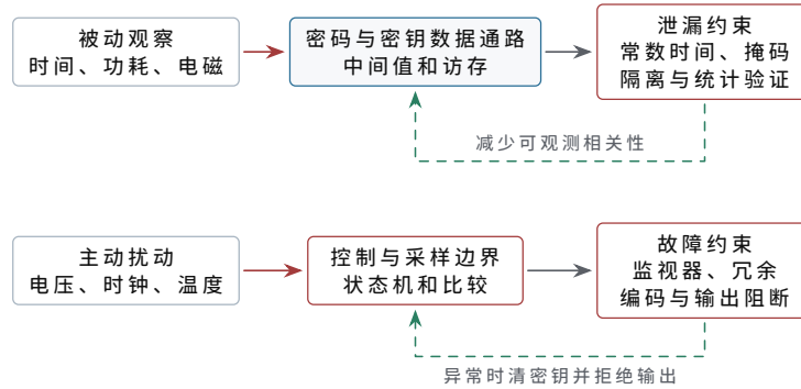
图示：侧信道与故障注入是两条相反的信息路径。侧信道从正常计算泄漏相关量，措施要降低“秘密-观测”的统计关系；故障注入从外部改变内部状态，措施要在结果发布前检测异常并阻断输出。两类措施不能互相替代。
