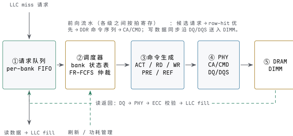
图示：内存控制器内部流水线。请求队列按 bank 组织（深度 8~32）；调度器查 bank 状态表选 row-hit 请求（FR-FCFS）；命令生成器把请求翻译成 DDR 命令序列并插入 ECC；PHY 驱动 CA/DQ/DQS 信号。
