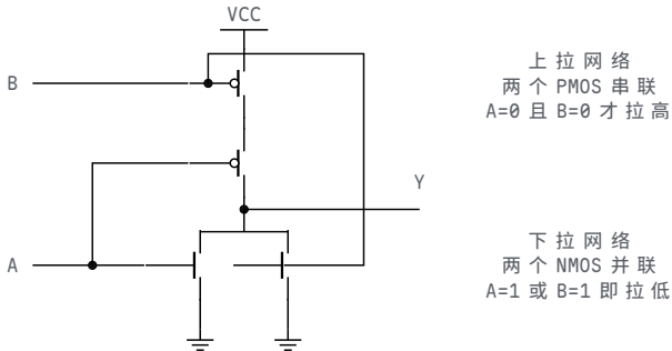
图示：二输入 NOR 的晶体管级结构，与上一张 NAND 图成对：上拉网络换成两个 PMOS 串联，只有 A=B=0 时上拉路径才完整、输出被拉到高；下拉网络换成两个 NMOS 并联，A 或 B 任一为 1 就有一条下拉路径把输出拉低。输出为 1 的唯一稳定条件对应“上拉串联路径完整”，与互补网络表逐行对应。（输入 B 的连线跨过输出线但不连接：没有连接点的交叉不算接通。）
