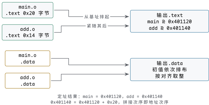
图示：静态链接的地址形成（对应正文 main.o 与 add.o 的最小例）。链接器把各输入文件的同类节依次拼接成输出的节： main.o 的 .text (0x20 字节) 铺在基址 0x401120 ， add.o 的 .text (0x14 字节) 紧随其后从 0x401140 开始；数据节同样处理。拼接完成，每个符号的值便从“节内偏移”换算成“节基址加偏移”的具体数— main = 0x401120 ， add = 0x401140 ，重定位所需的 S 至此全部就位。
