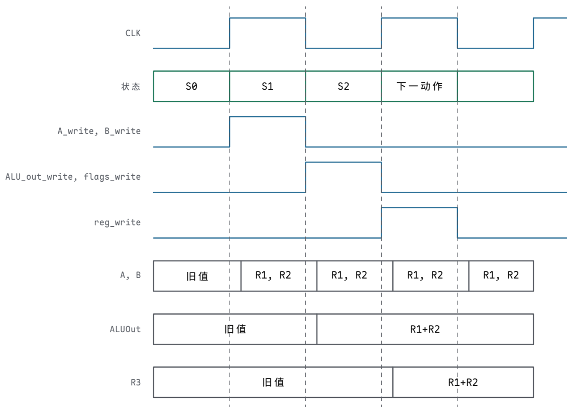
图示：三周期 R3=R1+R2 的对齐波形：控制线只在规定周期为高；状态元件只在上升沿提交。注意三条控制线的互斥关系——任何一拍 reg_write 提前变高，R3 都会被未成熟的价值污染；任何一拍 ALU_out_write 忘记关闭，ALUOut 锁存器就会混入旧值。
