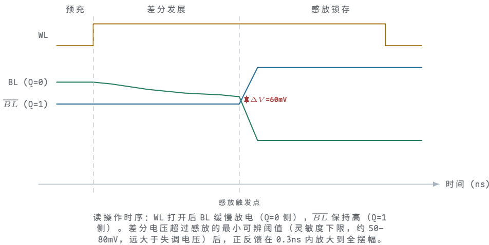
图示：SRAM 读操作波形。注意读操作是 非破坏性 的一读 Q=0 侧时 P1 栅接 \overline{Q}=VDD 处于截止，只要 N1 相对 M5 足够强（ CR > 1 ），Q 就不会被抬过翻转点，读完后单元数据不变。
