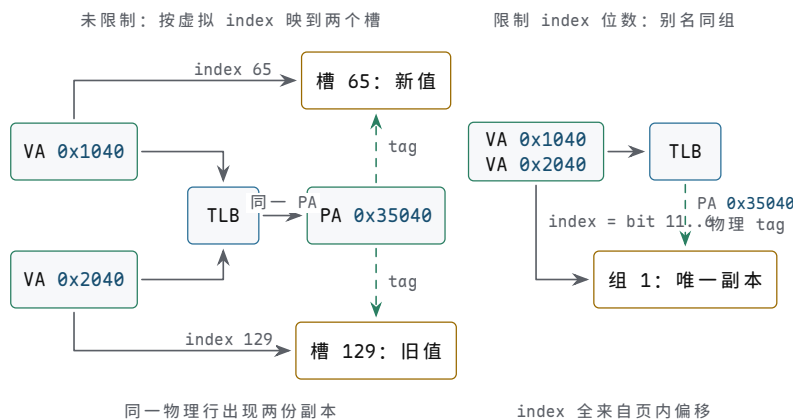
图示：VIPT 别名问题与限制 index 位数的对照。左：32 KiB 直接映射 cache 的 index 取 bit 14..6，0x1040 与 0x2040 的 index 分别是 65 与 129，同一物理行 0x35040 被存进两个槽，经 0x1040 写入后槽 65 是新值、槽 129 仍是旧值。右：限制 index 加 offset 不越出页内偏移 12 bit（如 32 KiB、8 路组相联，index 为 bit 11..6），两个别名的 index 都来自页内偏移，必然映到同一组，再由物理 tag 确认身份，双副本无从产生。
