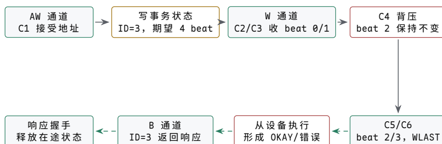
图示：一笔 AXI 写的状态链。地址接受、每个 data beat 接受、从设备执行和 B 响应握手是四类不同边界；C4 背压只延长 beat 2 的停留时间，不产生任何状态推进。
