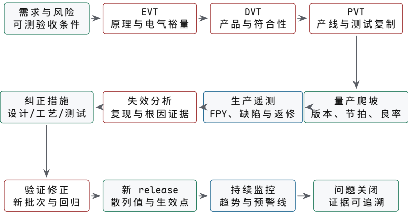
图示：从需求到量产问题关闭的三层闭环。EVT、DVT、PVT 是逐步扩大的验证阶段；量产数据又把真实缺陷送回失效分析。临时返修只有进入受控设计、工艺或测试 release，并由新批次验证后，才成为可复制的纠正措施。
