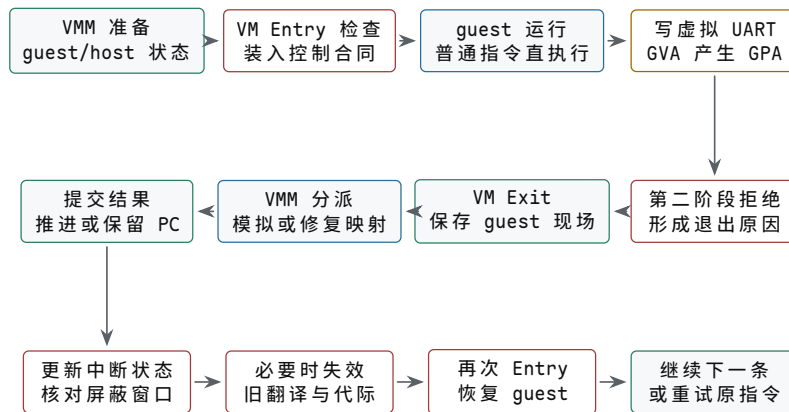
图示：一次由模拟 MMIO 触发的 VM Exit/Entry 闭环。上排从控制合同进入 guest，中排在第二阶段翻译处形成精确退出并交给 VMM，下排处理虚拟中断、翻译代际和再次进入。VMM 若完成指令模拟就推进 guest PC；若只是补映射等待原指令重试，则保留 PC。
