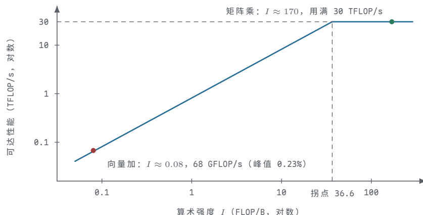
图示：双对数坐标下的 roofline：斜段是带宽屋顶（可达性能 = 带宽 × 算术强度），平段是算力屋顶 30 TFLOP/s，拐点 I^* = 30000/820 \approx 36.6 FLOP/B。向量加的强度只有约 0.08 FLOP/B，被带宽屋顶压在 68 GFLOP/s—峰值的 0.23%；矩阵乘约 170 FLOP/B，远在拐点右侧，峰值真正用满。横轴每往左一格，同样的算力折扣再重一倍。
