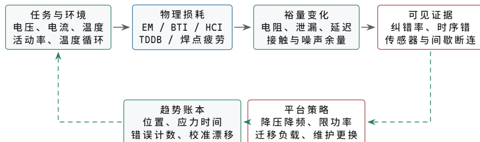
图示：老化不是一次离散故障，而是“应力积累-物理损耗-裕量下降-症状出现”的慢通路。平台只能观测传感器、错误计数和校准漂移等代理量，再通过降额或维护减少后续应力；恢复一次错误不会把已经消耗的材料寿命恢复到初始状态。
