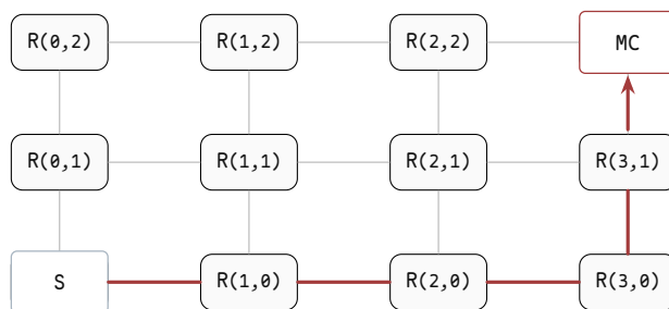
图示：4×3 Mesh 中从 S 到 MC 的唯一 XY 路径：先沿底行向右三跳，再沿最右列向上两跳。灰线表示其他可用链路，红线只表示本请求占用的五跳路径；图没有把返回包画成同一条反向箭头，因为响应使用独立虚拟网络和独立 credit。
