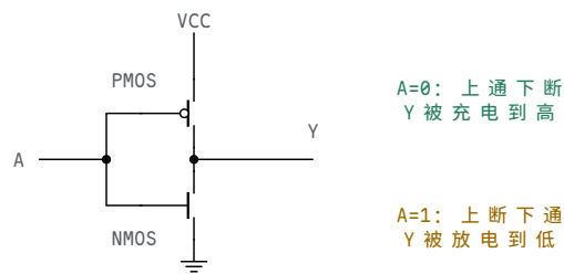
图示：反相器的开关模型。输入 A 同时接到两个控制端：PMOS 控制端带小圆圈，表示“输入低才导通”；NMOS 没有圆圈，表示“输入高才导通”。这就是 NOT 的全部——但它同时完成了二极管做不到的事：不管输入边沿多差，输出都被重新驱动成强 0 或强 1，电平被恢复了。
