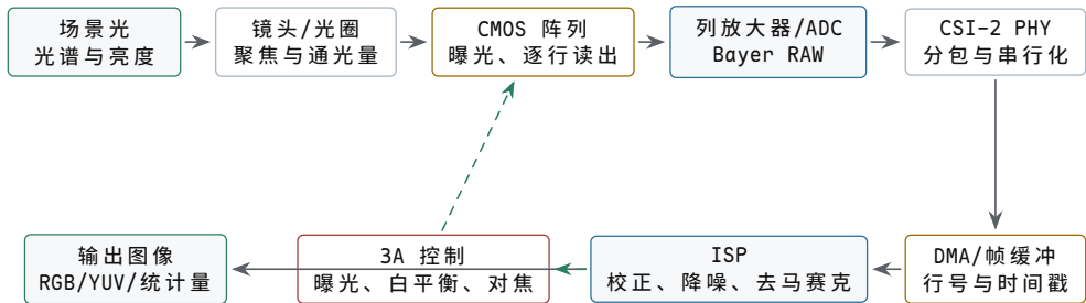
图示：相机数据面与控制面的闭环。上排把光转换成 Bayer RAW 并送入 CSI-2，下排由 DMA 和 ISP 生成图像；ISP 统计量还会驱动自动曝光、自动白平衡和自动对焦，修改下一批帧的传感器与镜头参数。一次控制调整通常要过若干帧才完全可见。
