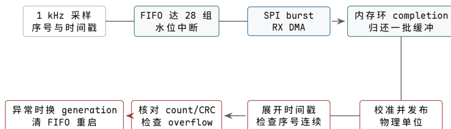
图示：物理时间由采样端记录，DMA completion 只说明一批字节已经进入内存。驱动按序号、FIFO 状态和时间戳恢复事件顺序；发现溢出或帧失步时，必须终止旧批次并从新 generation 重新建立时间关系。
