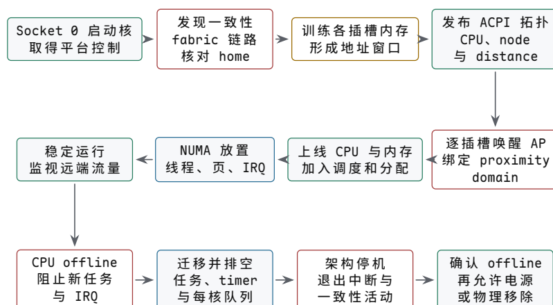
图示：双插槽平台从发现到退出的三层闭环。上排先让一致性 fabric、内存地址窗口和固件拓扑相互一致，中排才发布远端 CPU/内存供调度与分配使用，下排按上线所有权的逆序下线 CPU。逻辑 offline 完成后，平台还要满足机箱、电源和固件条件，才可能物理移除。
