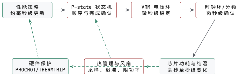
图示：DVFS 由多个时间尺度的控制器嵌套组成。P-state 状态机协调 VRM 与时钟的微秒级动作，热管理在更慢尺度上根据功耗和温度继续修正策略；PROCHOT/THERMTRIP 等硬件保护不等待软件环完成。
