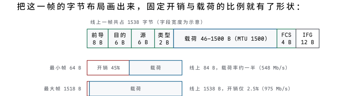
图示：以太帧在线上的字节布局：前导与 SFD 8 字节用于时钟锁定，MAC 地址与类型字段 14 字节，载荷最多 1500 字节，FCS 4 字节校验，帧间还有 12 字节静默。每帧 38 字节的固定开销与帧长无关：64 字节小帧把它摊成 45% 的负担，1518 字节大帧只付 2.5%—压力测试用小帧考 pps、吞吐测试用大帧考带宽，原因就在这张图上。
