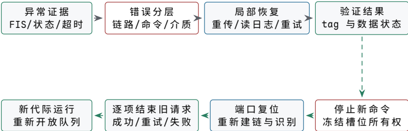
图示：错误恢复先尝试与失败层匹配的局部动作；只有错误持续或端口状态不再可信时，才冻结队列并复位端口。复位后仍要逐项处理旧 tag，再建立新代际并开放请求，不能把“链路重新起来”直接等同于所有旧命令都失败或都成功。
