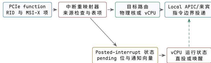
图示：MSI 消息经过来源绑定后才成为可投递中断。物理目标走上排进入 Local APIC；虚拟目标可在 posted-interrupt 状态中设置 pending 位，vCPU 正在运行时直接通知，未运行时先唤醒调度路径。两条路径都不能绕过 requester identity 与表项权限。
