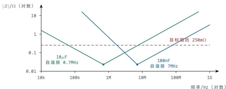
图示：PDN 阻抗随频率的分布（双对数示意）。单只电容的阻抗呈 V 形：低频端按 1/(2\pi fC) 下降，自谐振点触底，高频端被 ESL 接管按 2\pi fL 上升。两种容值的 V 形错开接力，设计目标是让合成阻抗在全频段压在目标线以下。
