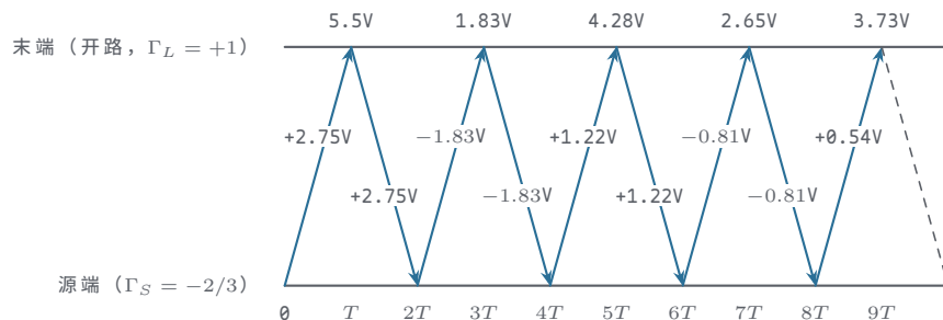
图示：弹跳图：横轴时间、纵轴位置，斜线是行波在源端与末端之间的来回，每跨一次耗时 T 。入射 +2.75\text{V} 在 t = T 到达开路末端， \Gamma_L = +1 全反射，末端跳到 5.5V；回波在源端按 \Gamma_S = -2/3 反号弹回，每往返一圈幅度乘 2/3 。上轨标出的各时刻末端电压 5.5、1.83、4.28、2.65、3.73V 与上表逐项一致，逐拍收敛到稳态 3.3V。
