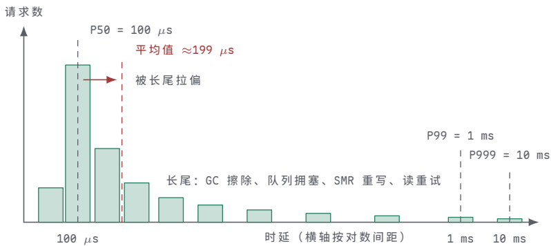
图示：消费级 NVMe SSD 4 KB 随机读的时延分布（横轴按对数间距）。主峰在 P50 = 100 \mu s；GC 擦除、队列拥塞、SMR 重写、读重试这类不常发生、一发生就是十倍百倍慢的事件，把分布拖出长尾：P99 = 1 ms，P999 = 10 ms。平均值被长尾向右拉偏，离中位数越来越远——所以外设时延必须带百分位一起报。
