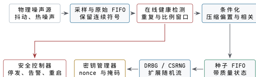
图示：随机数通路的两个完成域。健康检测通过只说明当前窗口未观察到规定异常；种子还要经过条件化并带质量状态进入 DRBG。健康检测失败时，控制器停止向密钥消费者提供新熵，而不是继续输出看似随机的数据。
