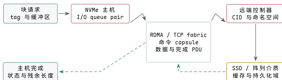
图示：一笔 NVMe-oF I/O 的三个所有权域。主机队列发布请求，fabric 只负责按 RDMA/TCP 契约传递命令和数据，远端控制器才解释命名空间并访问介质。网络 ACK、RDMA completion 和 NVMe CQ completion 属于不同层级；只有最后一项能结束 NVMe 命令，持久化还要满足 FUA/Flush 语义。
