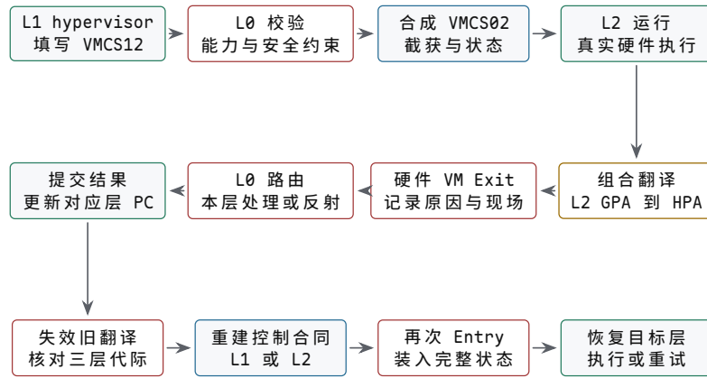
图示：L2 的一次进入、退出与恢复。VMCS12 是 L1 的控制意图，VMCS02 才是 L0 合成后交给硬件的执行合同。退出先回到 L0；L0 根据截获归属决定本层处理，还是构造等价现场反射给 L1。三层映射任一世代变化，都可能要求失效组合翻译。
