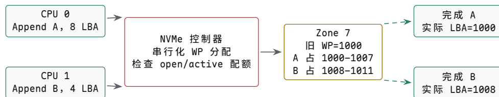
图示：同一 zone 上的两笔 Zone Append。控制器把“选择实际 LBA 与推进写指针”做成一个原子分配动作；完成项返回的位置才是上层可以提交到索引的地址。若 A 的完成晚于 B，上层仍按各自 CID 和返回 LBA 建立映射，不能按完成先后重新排列数据身份。
