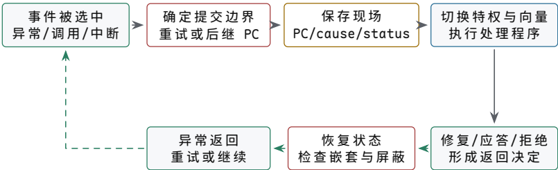
图示：陷阱的闭环由两条路径组成：上排在一个可恢复边界保存架构状态并进入处理程序；下排先消除或确认事件，再恢复状态并选择重试故障指令或从后继 PC 继续。返回指令提交之后，旧特权上下文才重新拥有执行权。
