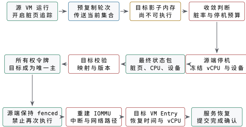
图示：一次预复制实时迁移。目标影子内存存在所有权交接前不能运行；停机窗口内发送最后脏页和不可并发复制的状态。令牌交接后源端必须保持 fenced，目标端重建 DMA、中断、网络和时间状态后才允许 VM Entry。
