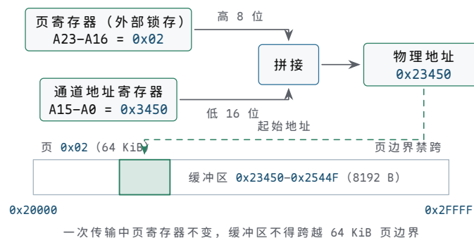
图示：8237 的 24 位地址拼接：外部页寄存器锁存 A23-A16，通道地址寄存器提供 A15-A0。示例页号 0x02、页内
