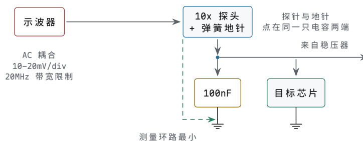
图示：纹波测量的标准接法。示波器切 AC 耦合挡住直流分量，用 10–20mV/div 的档位把纹波展开；10× 探头配弹簧地针，探针与地针直接点在同一只电容的两端——测的是负载端真实看到的电源，探头围出的测量环路也最小；示波器若有 20MHz 带宽限制就打开，挡住与电源无关的高频拾取。
