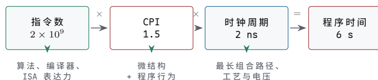
图示：程序时间三因子连乘：指令数由算法、编译器与 ISA 决定，CPI 由微结构与程序行为共同决定，时钟周期被最长组合路径封顶。数值取自本节的完整演算： 2 \times 10^9 条 \times 1.5 \times 2 ns = 6 s。任何优化手段都要先说清动的是哪个因子、另外两个动不动。
