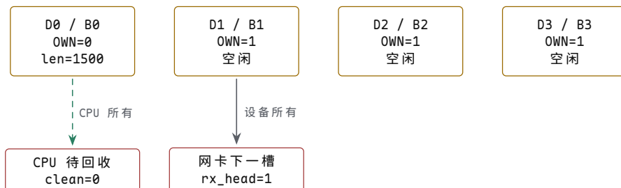
图示：网卡完成第一帧后的四槽环快照。四个描述符从左到右构成环的槽位顺序；D0 已交回 CPU，实际长度为 1500 B，D1-D3 仍归设备。网卡 head 已推进到 D1，但 D0 在驱动清理状态并重新发布 OWN 之前不能再次接收数据。
