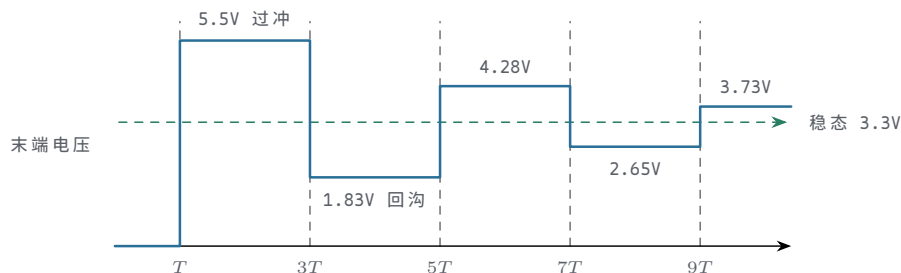
图示：3.3V、50Ω 走线、源阻 10Ω、末端开路时的末端电压逐拍演算。入射 2.75\text{V} 在 t = T 到达末端并全反射成 5.5V，回波在源端被负反射后逐拍抵消，每往返一圈幅度乘 2/3 ，最终收敛到稳态 3.3V。
