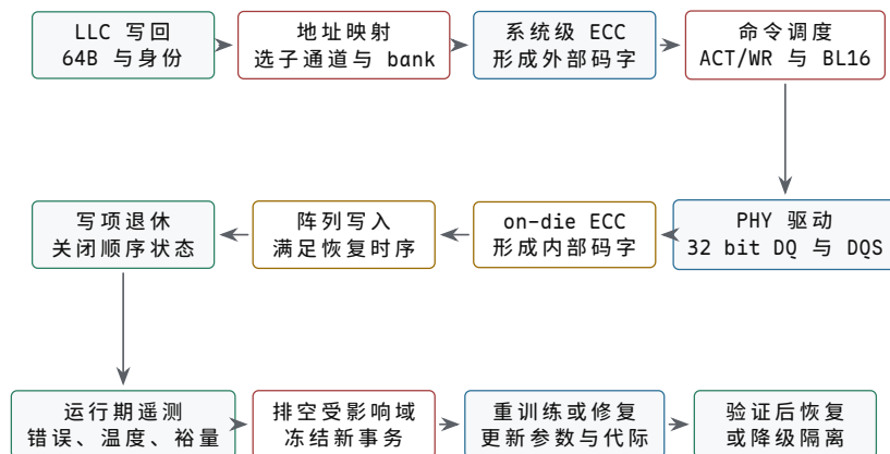
图示：DDR5 写入与运行期恢复的三层状态链。上排形成子通道可见的外部码字，中排完成 32 bit、BL16 数据突发和芯片内部编码，下排处理运行期裕量下降。on-die ECC 位不会出现在系统内存总线上；系统级 ECC 与器件内部 ECC 分别保护不同故障域。
