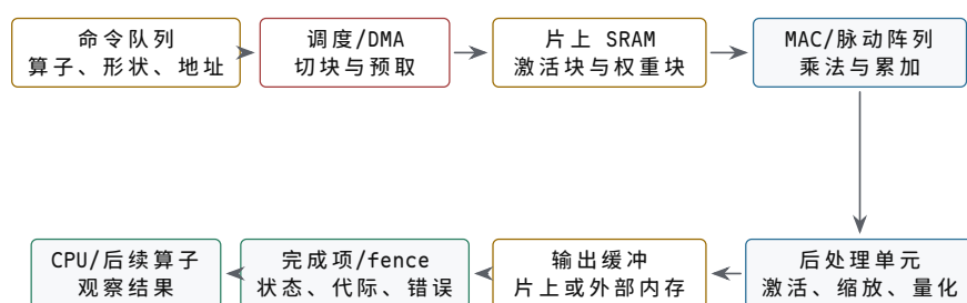
图示：一次 NPU 算子的请求-数据-完成闭环。调度器把大张量切成片上 SRAM 能容纳的块，MAC 阵列反复复用这些数据，后处理单元再完成激活与量化。输出写回、错误状态和 fence 必须按规定顺序发布，峰值 TOPS 不包含这些搬运与完成成本。
