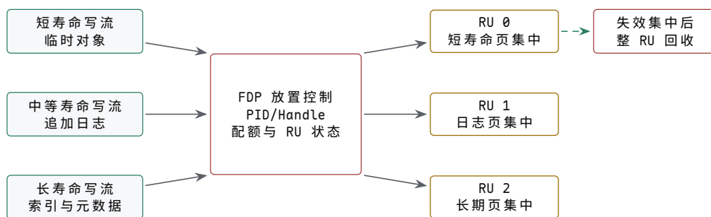
图示：FDP 的作用位置。主机只为写流附加寿命或租户维度的 placement，控制器仍拥有逻辑到物理映射；当短寿命数据集中失效时，RU 可以少搬或不搬长期数据便完成回收。完成项仍按普通 NVMe 队列返回，放置成功不等于数据已经持久化。
