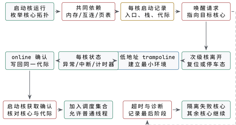
图示：一次次级核心上线事务。主路径从启动核发布记录、唤醒次级核，经过 trampoline 与每核初始化后返回 online 确认；只有启动核以匹配的 generation 获取确认后，调度器才使用该核心。虚线是超时分支，失败核心可以保持 offline，而不必让所有已健康核心一起停机。
