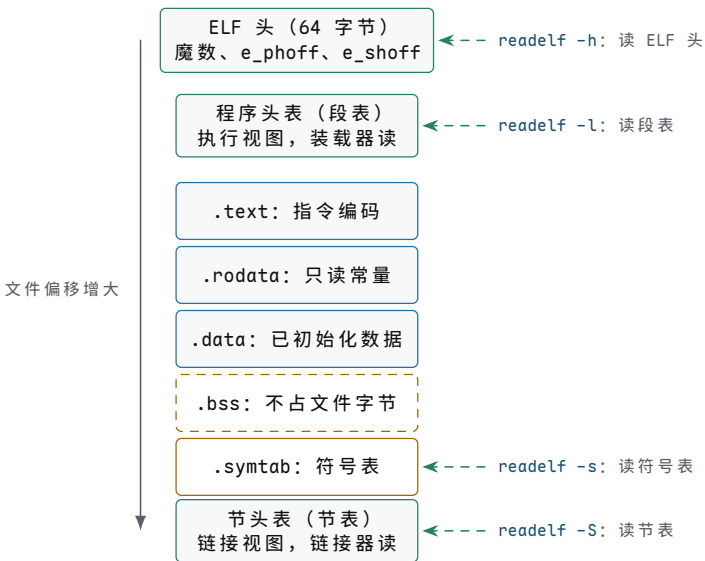
图示：ELF 文件按字节偏移的排布（自上而下偏移增大）。ELF 头中的 e_phoff 与 e_shoff 分别给出段表与节表的文
