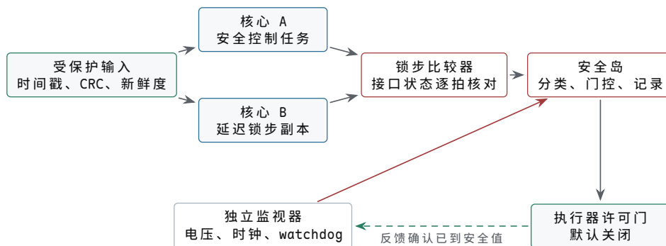
图示：锁步系统的责任边界。两个核心只提供分歧证据；安全岛还接收独立电压、时钟和 watchdog 证据，并控制默认关闭的执行器许可门。许可门反馈确认后，故障反应才完成。
