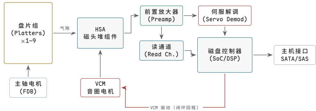
HDD 信号通路：磁头感应磁场 → 前置放大 → 读通道（均衡+Viterbi+LDPC）→ 控制器 → SATA/SAS → 主机。伺服路径：Preamp → Servo Demod → Controller → VCM Driver → VCM。写路径反向：Controller → Write Channel → Preamp → 磁头。
