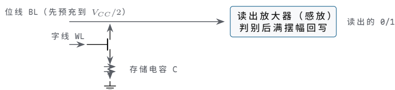
打开字线后，电容与位线共享电荷，位线电压轻微上升或下降；感放判别方向输出 0/1，并立刻把满摆幅电平写回单元——读出即重写。
