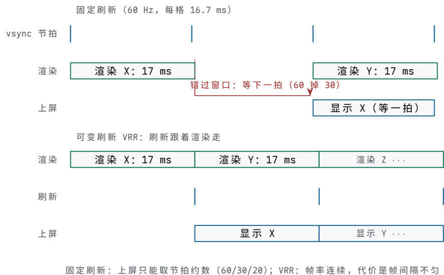
图示: 固定刷新与可变刷新的帧时序对照 (横轴每格约 16.7 ms)。上方固定刷新: 交换只能发生在 vsync 窗口, 渲染耗时 17 ms、比预算多 0.3 ms, 完成时刻错过当拍窗口, 只能对齐到下一拍—帧率从 60 直接掉到 30, 中间没有任何档。下方 VRR: 显示器不再按固定节拍催帧, 等 GPU 宣布帧就绪才扫下一帧, 17 ms 的帧按约 59 Hz 显示, 帧率第一次可以连续变化; 代价是帧间隔忽长忽短, 低到面板下限以下时靠倍帧补偿。
