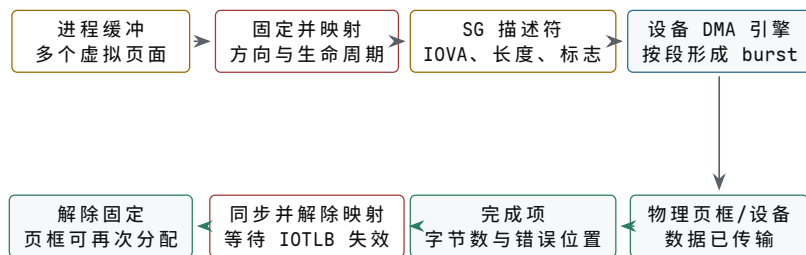
图示：Scatter-gather 的提交与回收闭环。上排把离散页框固定、映射并编码为设备可读的段列表；下排只有在设备完成、CPU 重新获得可见性且 IOMMU 旧翻译失效后，页框才可解除固定并复用。
