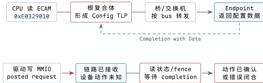
图示：配置读和运行期写具有不同完成语义。配置读必须取得带 tag 的 completion；运行期 posted MMIO write 没有逐笔 completion，驱动若需要确认设备副作用，必须使用设备规定的状态读、flush 或 fence。
