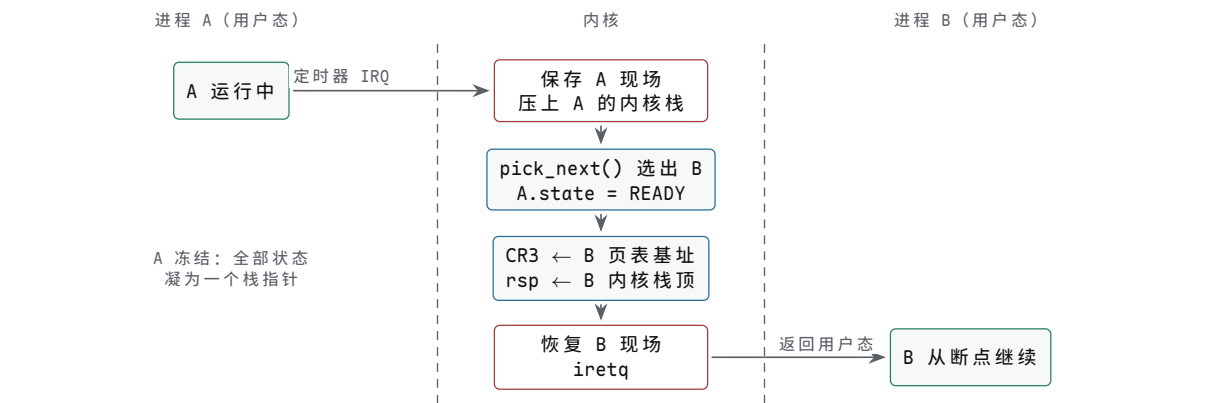
图示：上下文切换泳道（对应正文 trace）。定时器中断在指令边界把 CPU 从 A 带进内核：A 的现场压上它自己的内核栈，调度器选出 B 后写入 B 的页表基址（CR3）、把栈指针切到 B 的内核栈，再弹出 B 的寄存器并 iretq —返回落进 B 的用户态，B 只得上次陷入返回得特别久。被切走的 A，全部状态归结为进程控制块里的一个栈指针，等下次被选中时原路恢复。
