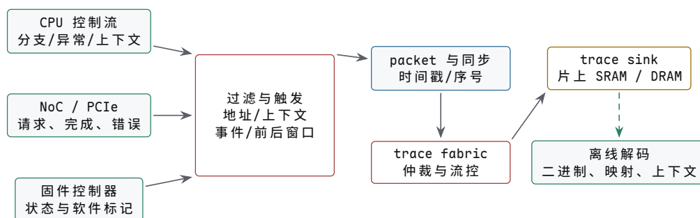
图示：片上 trace 是一条与被测数据通路并行的证据通路。source 产生事件，过滤器限制流量，fabric 把多个时钟域的 packet 送到 sink，解码器再结合外部映射还原语义。任何一级溢出或缺少同步标记，都会使后续证据出现
