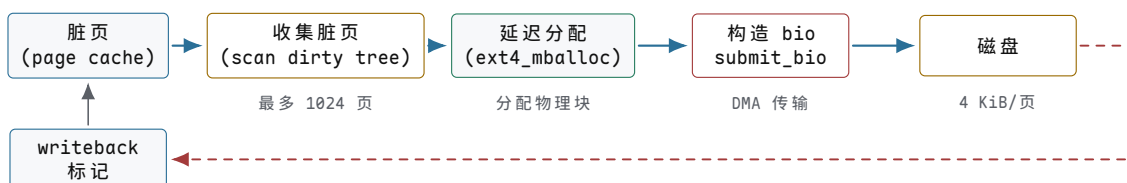
图示：写回数据流。脏页从 page cache 出发，经过脏页扫描、延迟分配、bio 构造、DMA 传输到达磁盘。I/O 完成后中断回调清除 writeback 标记，page 变为干净页留在 cache 中。
