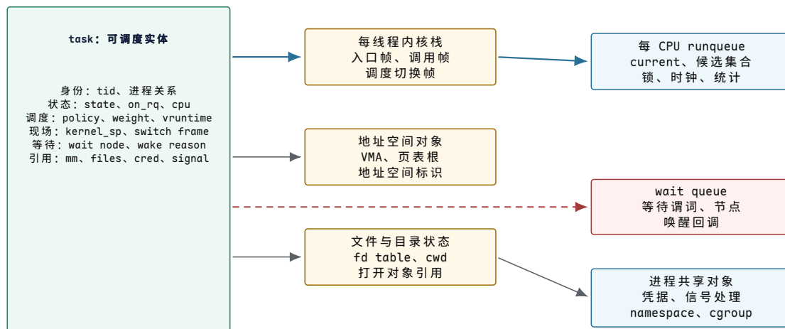
图示: task 不是“进程全部资源的盒子”。它保存恢复执行和参加调度所需的私有状态，并引用地址空间、文件表和安全状态。运行时， task 由某个 CPU 的 current 到达；阻塞时，由等待队列节点到达；两种位置必须互斥。
