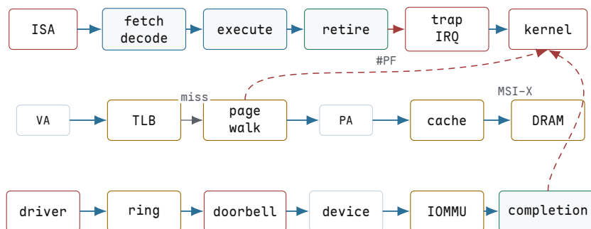
图示：三条关键链：CPU 提交链、地址翻译与 cache 链、设备 DMA 链。OS 必须把它们的状态边界对齐。
