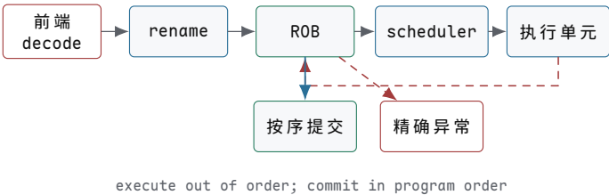
图示：乱序 CPU 的教学结构。rename 和 scheduler 提高并行度，ROB 保证 precise exception 和按序提交。
