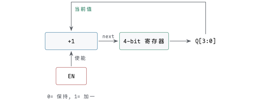
图示：4-bit 同步计数器。
