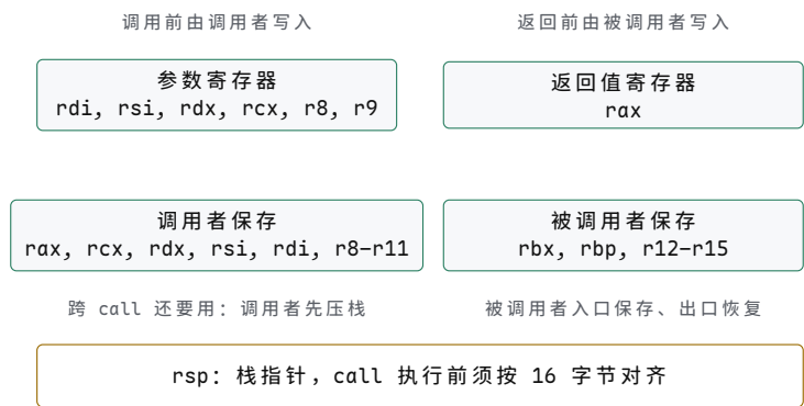
图示：System V AMD64 调用约定的寄存器分工。前 6 个整型参数依次进入 rdi 、 rsi 、 rdx 、 rcx 、 r8 、 r9 ，返回值进入 rax ；调用者保存寄存器跨 call 不保证保持，还需要旧值时由调用者自己压栈；被调用者保存寄存器由被调用者在入口保存、出口恢复。本章 sum2 的参数 edi/esi 、返回值 eax 和序言里的 push rbx ，正是按这张图分工的实例。
