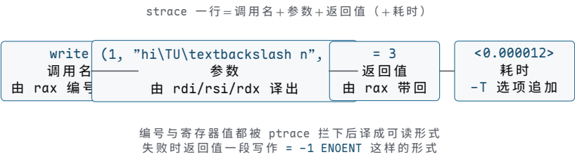
图示：典型 strace 行的字段分解（调用行与正文 write(1, "hi\\TU\\textbackslash n", 3) = 3 一致）。 strace 借 ptrace 在每次陷入与返回时拦一下：陷入时读 rax 译出调用名、读 rdi/rsi/rdx 译出参数，返回时读 rax 译出返回值——出错则印成 = -1 ENOENT 加一行说明；耗时一段只有加 -T 才出现在行尾（图中数值为示例）。一行的四段，全部来自“系统调用与异常控制流”一节那条 ABI 约定里的寄存器。
