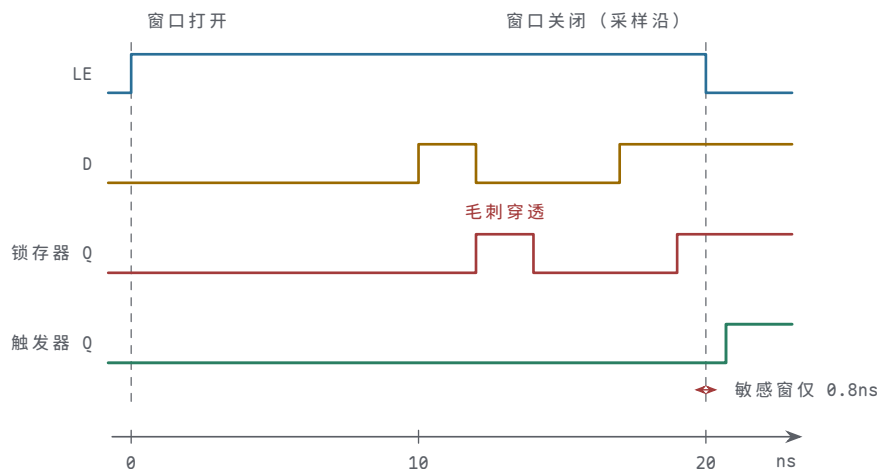
图示：同一个 D 送到两种元件：LE 窗口 ( t=0 到 20\text{ns} ) 内， D 上 2\text{ns} 宽的毛刺 ( t=10\text{ns} ) 和晚到的变化 ( t=17\text{ns} ) 都经过约 2\text{ns} 延迟穿透到锁存器 Q ； D 触发器只认 t=20\text{ns} 采样沿前后共 0.8\text{ns} 的窗口，毛刺完全不可见，晚到变化被正常采入，沿后 Q 一步更新。敏感区 20\text{ns} 对 0.8\text{ns} ，相差 25 倍——这就是透明窗口的代价。
