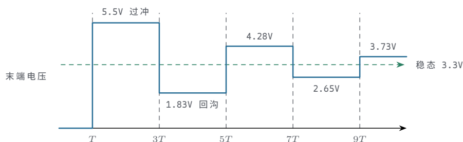
图示：3.3V、50Ω 走线、源阻 10Ω、末端开路时的末端电压逐拍演算。入射 2.75\text{V} 在 t = T 到达末端并全反射成 5.5\text{V} ，回波在源端被负反射后逐拍抵消，每往返一圈幅度乘 2/3 ，最终收敛到稳态 3.3\text{V} 。
