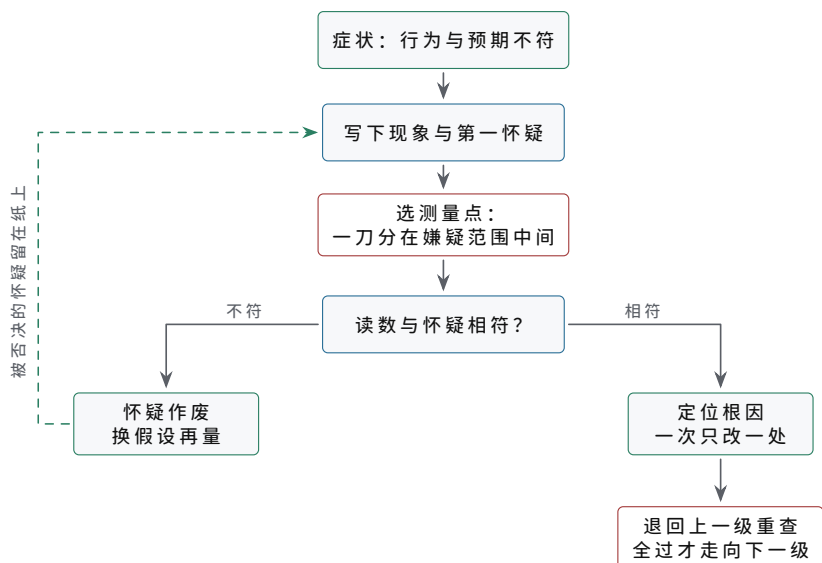
图示：故障排查决策树（对应联调日志六步的走法）。症状写下后提出第一怀疑，怀疑的职责是指定第一个测量点——选在与各嫌疑都无关、一刀分在范围中间的位置量；读数与怀疑不符，怀疑就地作废、换假设再量；相符才动手，一
