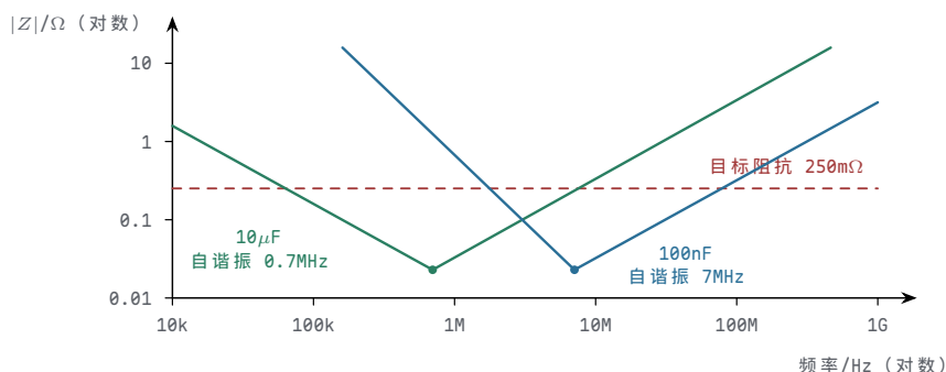
图 20-1 PDN 阻抗随频率的分布（双对数示意）。单只电容的阻抗呈 V 形：低频端按 1/(2\pi fC) 下降，自谐振点触底，高频端被 ESL 接管按 2\pi fL 上升。两种容值的 V 形错开接力，设计目标是让合成阻抗在全频段压在设计目标线以下。
