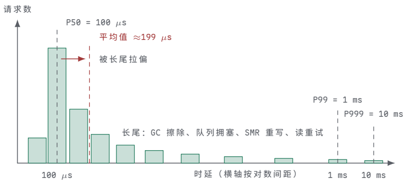
图示: 消费级 NVMe SSD 4 KB 随机读的时延分布 (横轴按对数间距)。主峰在 P50 = 100 \mu\text{s} ; GC 擦除、队列拥塞、SMR 重写、读重试这类不常发生、一发生就是十倍百倍慢的事件, 把分布拖出长尾: P99 = 1 \text{ ms} , P999 = 10 \text{ ms} 。平均值被长尾向右拉偏, 离中位数越来越远——所以外设时延必须带百分位一起报。
