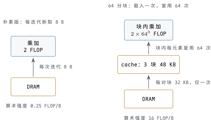
图示：同一段矩阵乘的两种数据流。左：朴素版内层每次乘加都从 DRAM 新取两个元素，2 FLOP 配 8 B，强度 0.25 FLOP/B，与矩阵规模无关。右： 64 \times 64 分块后三个块共 48 KB 驻留 cache，每对块从 DRAM 读入 32 KB 只有一次，块内完成 2 \times 64^3 次乘加——字节被反复使用，强度升到 16 FLOP/B。优化没有改动任何一次浮点运算，只改了字节走的路程。
