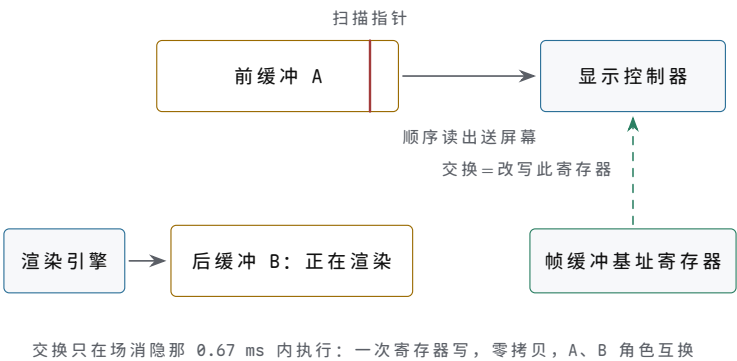
图示：双缓冲把渲染与扫描分开：渲染引擎写后缓冲 B，显示控制器经扫描指针读前缓冲 A，两块缓冲互不干扰。交换只是改写显示控制器的帧缓冲基址寄存器——一次寄存器写，零拷贝——且只在场消隐那 0.67 ms 内执行，此后 A、B 角色互换。只要交换点严格避开扫描窗口，撕裂从机制上消失，这就是垂直同步；若扫描中途改写基址，屏幕上半是旧帧、下半是新帧，即 tearing。
