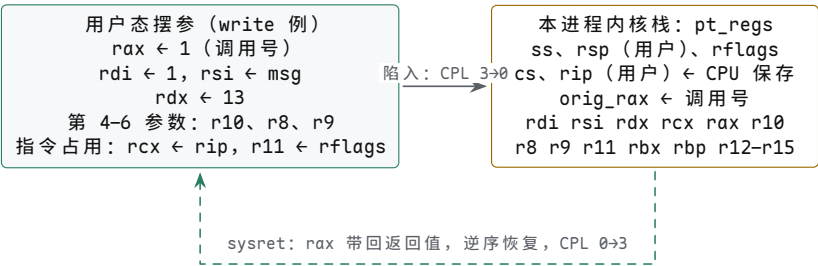
图示：系统调用的参数传递与现场保存 ( write(1, msg, 13) 例)。用户态按 ABI 摆好 rax 编号与 rdi/rsi/rdx 参数； syscall 指令把返回地址装进 rcx 、标志装进 r11 ——这正是第四个参数改用 r10 的原因——并把 rip 换成 LSTAR 入口。入口代码切到本进程内核栈，把用户态现场连同全部通用寄存器存成 pt_regs ，内核 C 代码看到的“寄存器”就是这张内存表； sysret 逆序恢复，返回值仍由 rax 带回，一进一出同一个寄存器。
