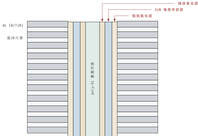
3D NAND 垂直截面：从沟道中心向外依次为 poly-Si 沟道 → 隧穿氧化层 → SiN 电荷俘获层 → 阻挡氧化层 → W/TiN 字线。每层字线与沟道交叉处形成一个存储单元。
