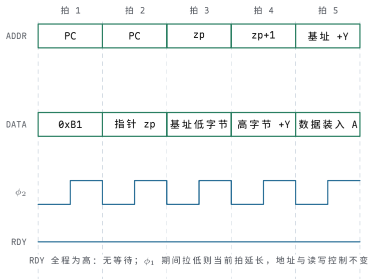
图示：LDA (zp),Y 的五拍总线时序：五拍全为读周期，每拍地址先送上总线，数据在 \phi_2 窗口内由存储器驱动，CPU 在 \phi_2 结束前采样。第 4 拍读基址高字节的同时，低字节与 Y 相加形成最终地址；RDY 全程为高，故没有任何等待
