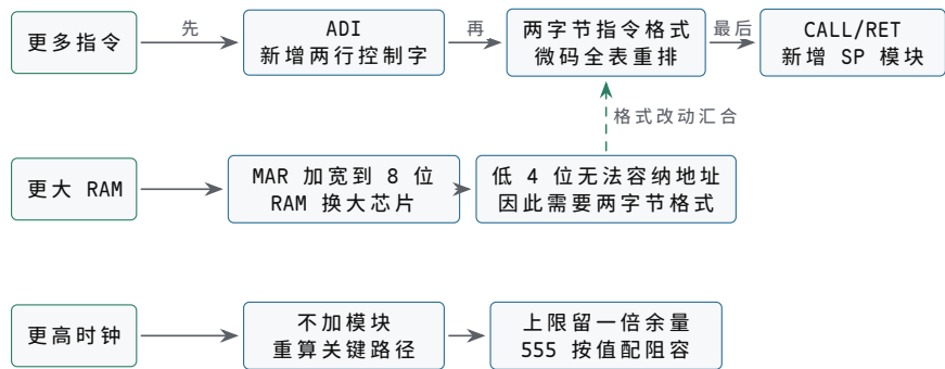
图示：扩展路径决策（对应正文扩展方向表）。三个目标各有相应的实现路径：加指令按成本递增排—ADI 只需新增两行控制字，成本最低；两字节指令格式要重排全表微码；CALL/RET 与栈需要新增 SP 计数器模块，成本最高。扩 RAM 连锁最多：MAR 加宽、RAM 换大之外，低 4 位无法容纳地址，因此同样需要两字节格式。提高时钟不加模块，只重算“总线到 ALU 到 A 建立时间”这条关键路径，理论上限再留一倍余量。所以扩展的顺序不是随机的：先有栈才谈得上子程序，再有富余的地址空间才谈得上中断向量。
