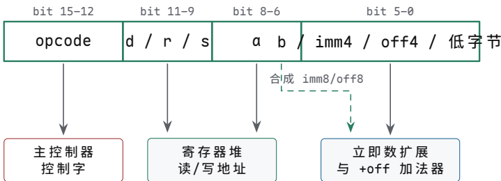
图示：16-bit 编码的字段条与各字段的译码去向。opcode 固定占 bit 15-12，第一级译码只接这 4 位；d/r/s 与 a 位置恒定，直接驱动寄存器堆的读/写地址，与 opcode 译码并行启动；低位段进入立即数扩展与偏移加法路径，长立即数 imm8/off8 由 a 字段与低位段合成（虚线）。以 0x7260 核对：高 4 位 0111 是 SHL，d=a=001，imm4=1000=8。 字段位置定下来之后，下面的数据通路图里那些从 IR 直接引出的线才有依据：寄存器字段到寄存器堆读地址的竖线、立即数扩展器的输入、偏移到 +off 加法器的路径，都对应这里的固定位置。
