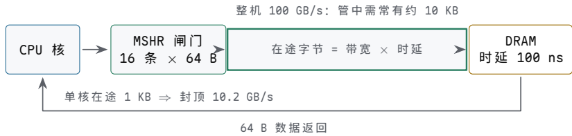
图示：Little 定律的直观版：时延 100 ns 的水管里要维持 100 GB/s，线上必须随时有约 10 KB 字节在途。单核的 MSHR 只有 16 条、在途预算 1 KB，于是单核带宽被闸门封顶在 1 KB/100 ns ≈ 10.2 GB/s—水管再粗，闸门只开这么宽。
