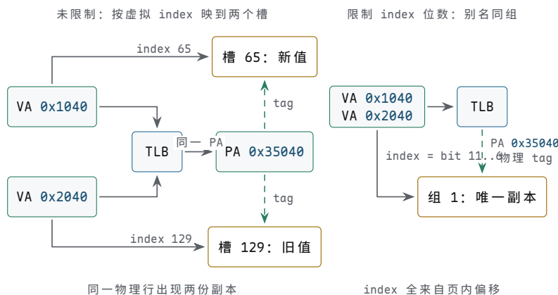
图示：VIPT 别名问题与限制 index 位数的对照。左：32 KiB 直接映射 cache 的 index 取 bit 14..6，0x1040 与 0x2040 的 index 分别是 65 与 129，同一物理行 0x35040 被存进两个槽，经 0x1040 写入后槽 65 是新值、槽 129 仍是旧值。右：限制 index 加 offset 不超出页内偏移 12 bit（如 32 KiB、8 路组相联，index 为 bit 11..6），两个别名的 index 都来自页内偏移，必然映到同一组，再由物理 tag 确认身份，双副本无从产生。
