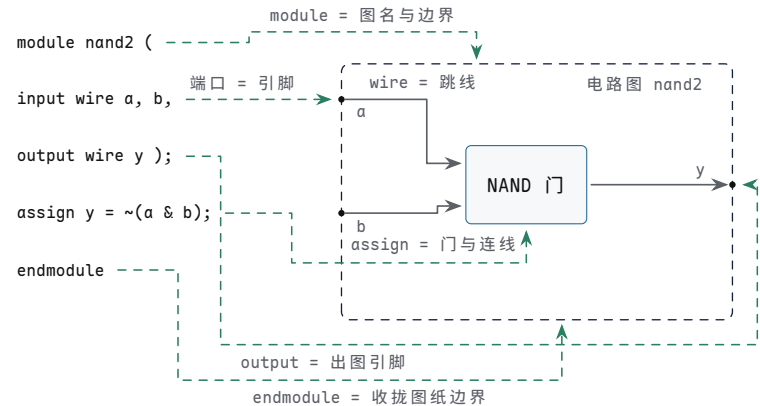
图示：这几行代码与电路图元的逐项对应（虚线为对应关系，不是电路连接）： module/endmodule 圈出图纸边界，端口表给出进出图的三根引脚， wire 是引脚到门之间的跳线， assign 把一只 NAND 门接在 a 、 b 与 y 之间。读任何 module 都用这个顺序：先看引脚，再数跳线，最后对每个门对号入座。
