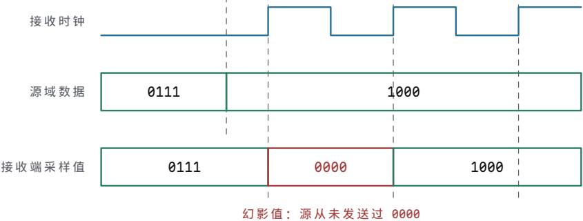
图示：4-bit 计数值从 0111 跳变到 1000，四个 bit 同时变化；各路两级同步器的走线和器件延迟略有差异，最高位的新值到得比低三位晚。接收端在 x=4 的采样沿采到低三位的新值和最高位的旧值，于是依次看到 0111、0000、1000——中间的 0000（红色）是源从未发送过的幻影值。逐级加触发器消除的是亚稳态，消除不了各位之间的采样时刻分歧；多 bit 跨域必须靠握手、格雷码或异步 FIFO 把数值作为整体传递。
