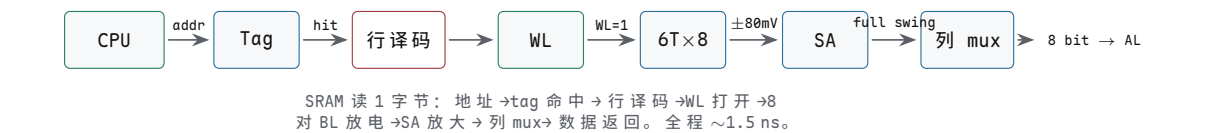
图示：SRAM 读路径。每一步都是组合逻辑或单级放大，没有等待状态，因此 L1 访问可以在一个时钟周期内完成。
