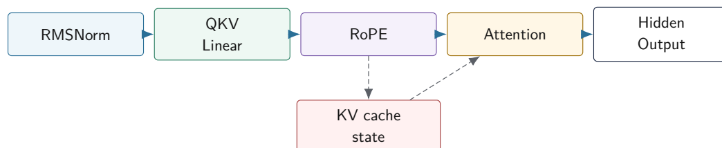
图示：本图要证明的命题是：Graph IR 不只记录张量数据流，还要显式记录 KV cache 这样的跨 token 状态边。
