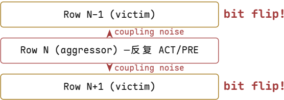
每次 ACTIVATE 激活 Row N 时，WL 电压从 0 跳到 VDD (boosted)，通过寄生电容耦合到相邻行的存储节点，使 victim 行电荷微量泄漏。累积足够多次后，victim 行数据翻转。
