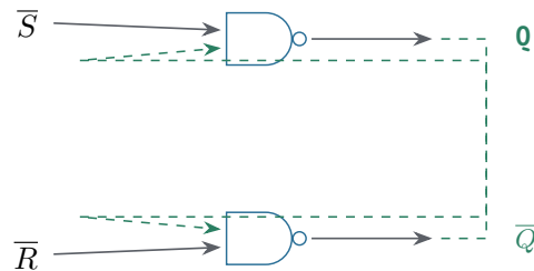
交叉反馈只连接到另一只 NAND 的第二输入, 输入线、输出线和反馈线各走独立通道。
