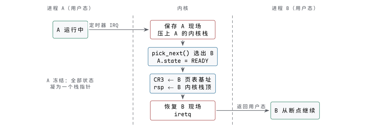
图示：上下文切换泳道（对应正文 trace）。定时器中断在指令边界把 CPU 从 A 带进内核：A 的现场压上它自己的内核栈，调度器选出 B 后写入 B 的页表基址（CR3）、把栈指针切到 B 的内核栈，再弹出 B 的寄存器并 iretq —返回落进 B 的用户态，B 只得上次陷入返回得特别久。被切走的 A，全部状态归结为进程控制块里的一个栈指针，等下次被选中时原路恢复。
