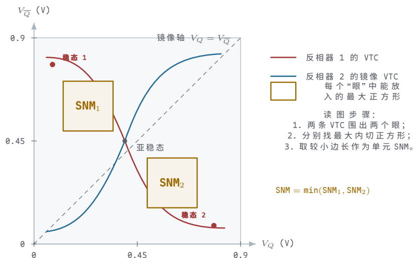
图示：SRAM 蝶形图与 SNM 测量。两个稳态点 (红点) 位于对角；亚稳态点 (灰点) 在中心。SNM 越大，单元越不容易被噪声翻转。
