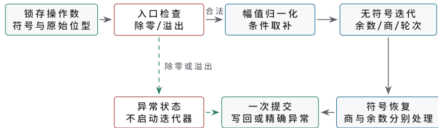
图示：有符号整数除法的控制闭环。上排只在入口合法时启动耗时的无符号迭代；下排把正常结果或异常送到同一个提交点。中间余数和部分商均是微架构状态，不能提前改变体系结构目标寄存器。
