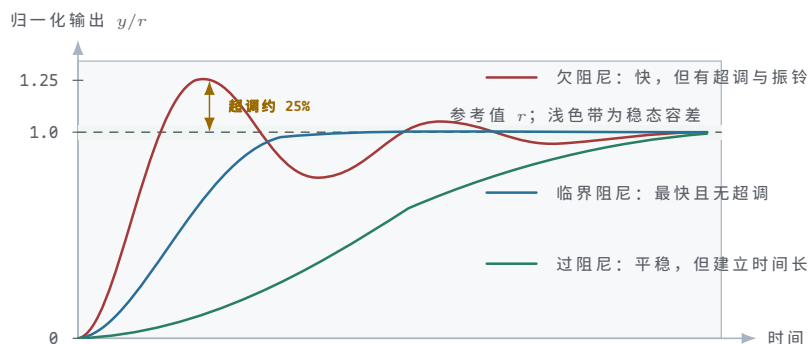
图示：同一阶跃目标下三种阻尼形态的响应。欠阻尼环（相位裕度小）上升最快，但冲过目标后振荡数次才停稳；过阻尼环（裕度大、带宽低）不越雷池一步，却慢得多；临界阻尼是不超调前提下最快的形态。工程上常故意留一点超调（相位裕度 45^\circ 上下，超调约 15%~25%），用少量振荡换取明显更快的响应。
