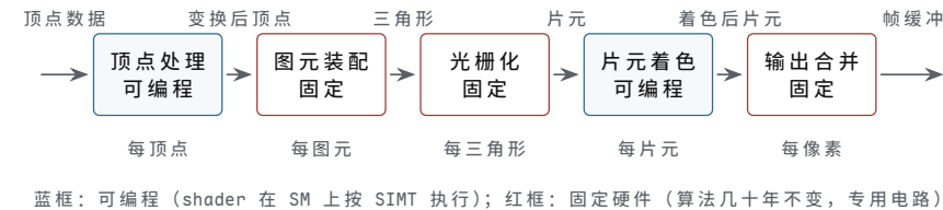
图示: 图形管线五阶段: 数据形态沿顶点、三角形、片元、颜色一路变换, 每一级的输出就是下一级的输入。可编程与固定的分界清清楚楚——顶点处理与片元着色交给 shader, 在 SM 上按 SIMT 跑; 装配、光栅化、输出合并的算法几十年不变, 做成固定电路。级间全走先进先出队列, 不需要全局调度者。
