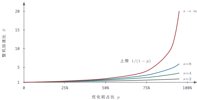
图示：Amdahl 定律的四条加速曲线。 s \rightarrow \infty 那条就是上限 1/(1-p) ， p = 0.9 时也只会到 10；其余三条被它压在下面。读法： s 决定曲线弯成什么形状， p 决定曲线能爬到多高一占比才是主变量。
