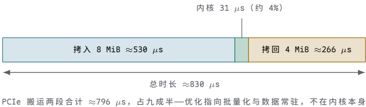
图示：一次内核启动的耗时构成 ( N = 2^{20} 向量加, PCIe 3.0 x16, 按比例)：拷入 8 MiB 约 530 \mu s，内核执行约 31 \mu s，拷回 4 MiB 约 266 \mu s，总时长约 830 \mu s。两次 PCIe 搬运占九成半，内核只占约 4%—算术强度约 0.08 FLOP/B 的负载，时间几乎全花在搬运上；工程上要么批量化、让数据常驻显存把这笔固定开销摊薄，要么干脆留在 CPU 上。
