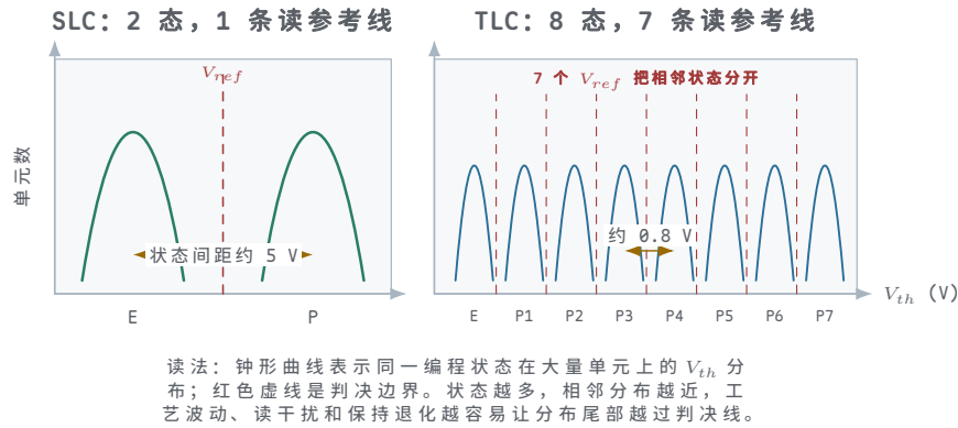
图示: SLC 与 TLC 的 V_{th} 分布对比。SLC 只有擦除态 (E) 和编程态 (P), 间距大 ( \sim 5V ), 抗干扰能力极强。TLC 有 8 个状态 (E, P1-P7), 相邻间距仅 \sim 0.8V , 需要 7 个读参考电压。QLC 有 16 个状态, 间距压缩到 \sim 0.4V 。
