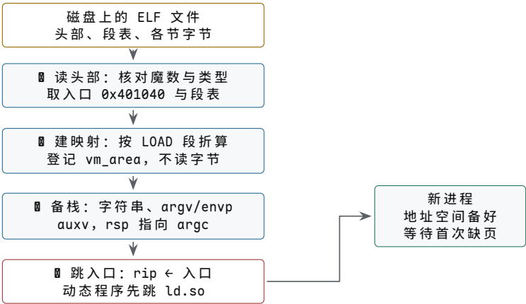
图示： execve 的四步流程（数值对应正文 hello 例）。内核核对魔数与类型后取出入口 0x401040 与段表，把每个 LOAD 段折算成一条映射登记下来——此时程序的一个字节都还没进内存；再把参数字符串、 argv/envp 与辅助向量摆上栈顶，最后设置 rip ：静态程序直指入口，动态程序先给动态链接器。四步几乎不搬数据，所以 execve 很快；失败时正常返回 -1 ，四步一件都没做。
