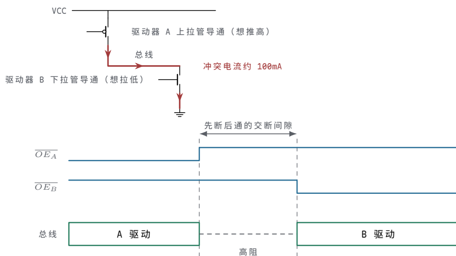
图示：上：两个三态驱动器同时使能时的冲突通路——电流从 VCC 经 A 的上拉管、总线、B 的下拉管直到 GND（图中只画出导通的管子，另一只方向的管子均关断），按每个输出级导通电阻约 25\Omega 估算约 100\text{mA} ，总线电平停在中点附近，既不是合法高也不是合法低。下：正确的驱动权交接——A 的使能先撤、输出进入高阻，留出先断后通的切换间隙后 B 才使能，任何时刻总线上最多一个驱动器。
