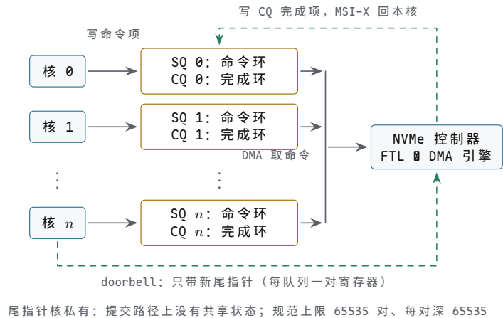
图示：NVMe 的多队列结构：每核一对 SQ/CQ，尾指针核私有，doorbell 只携带新尾指针；设备经 DMA 取走命令、写 CQ 完成项，再以 MSI-X 按队列分发回本核——提交与完成两条路径都不出核。免锁不是锁实现得好，而是提交路径上根本没有共享状态。规范允许最多 65535 对队列、每对深 65535，真实盘实现几十到几千对，常用深度 32 至 1024。
