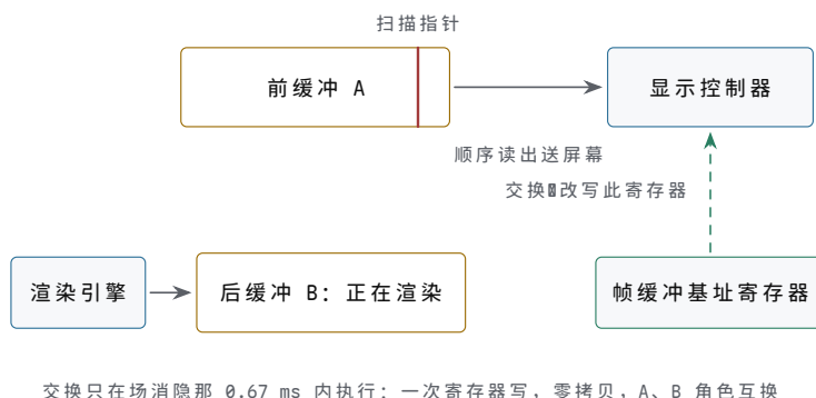
图示：双缓冲把渲染与扫描分开：渲染引擎写后缓冲 B，显示控制器经扫描指针读前缓冲 A，两块缓冲互不干扰。交换只是改写显示控制器的帧缓冲基址寄存器——一次寄存器写，零拷贝——且只在场消隐那 0.67 \text{ ms} 内执行，此后 A、B 角色互换。只要交换点严格避开扫描窗口，撕裂从机制上消失，这就是垂直同步；若扫描中途改写基址，屏幕上半是旧帧、下半是新帧，即 tearing。
