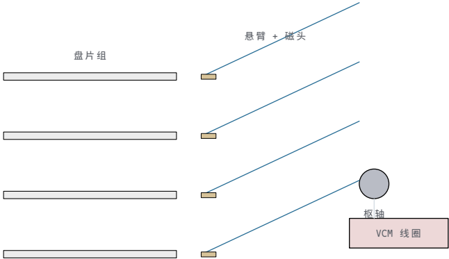
HSA 侧视：所有悬臂固定在公共枢轴上，VCM 驱动整个组件绕枢轴旋转。每个悬臂末端是滑块 + 磁头，通过柔性铰链 (flexure) 允许微量俯仰和偏转。
