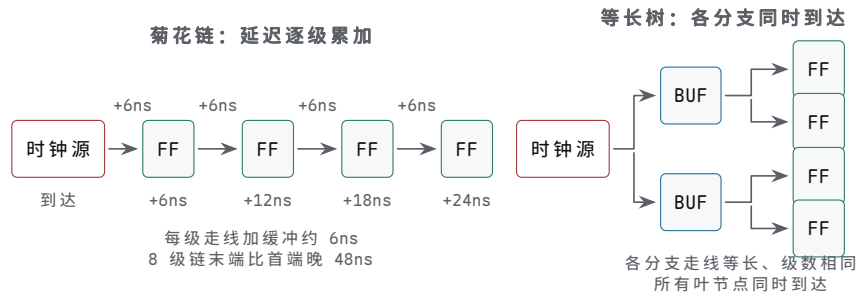
图示：时钟分配的两种结构。菊花链中每级走线与缓冲延迟逐级累加，末端沿越来越晚；等长树让每条“根到叶”路径的走线长度与缓冲级数相同，缓冲延迟在分支间相消，所有触发器在结构上同时看到时钟沿。
