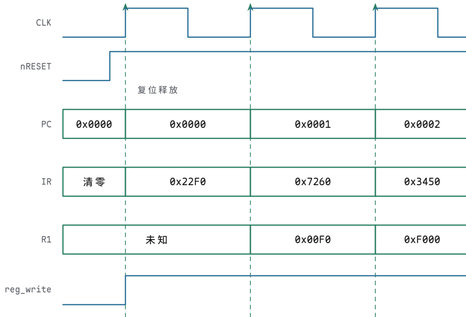
图示：复位后前三个周期的时序，对照 § 二 ROM 程序开头三条编码（ 0x22F0=MOV\ R1, 0xF0 、 0x7260=SHL\ R1, 8 、 0x3450=MOV\ R2, [R1+4] ）。复位把 PC 保持在 0x0000 、写使能保持在安全值；释放后每个周期内组合路径完成取指、译码、执行，周期末上升沿才提交新状态—— 0x00F0 在第二个上升沿、 0xF000 在第三个上升沿写进 R1。这张波形图直观展示了“状态只在时钟沿改变”，单步调试时应逐格核对。
