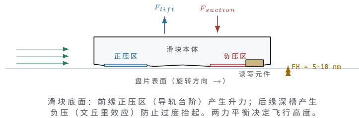
图示：滑块侧视（非等比例）。实际滑块尺寸 ~1.25 mm × 1.0 mm，飞行高度 5-10 nm，导轨台阶高度 ~50-200 nm。
