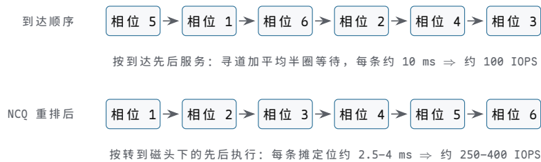
图示：同一批随机请求的两种服务顺序（示意六个，实际是 32 个在途）。按到达先后服务，相邻请求相位乱跳，每条都要付一次寻道加平均半圈的旋转等待；盘内固件知道磁头位置与盘片角度，按”当前柱面加旋转相位”重排后，同一柱面的请求按转到磁头下的先后执行，旋转等待被摊薄，每条定位约 2.5-4 ms。时延没变，在途数变了一IOPS 从约 100 提到约 250-400。
