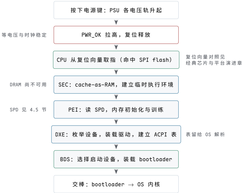
图示：UEFI 开机流程。前半段被硬件约束主导：电压与时钟稳定之前不能释放复位，内存训练完成之前只能用 cache 充当内存；后半段被软件结构主导：驱动按依赖调度，表建好后才交棒。任何一步失败，整机表现为“点不亮”，而根因可能远在 CPU 之外。
