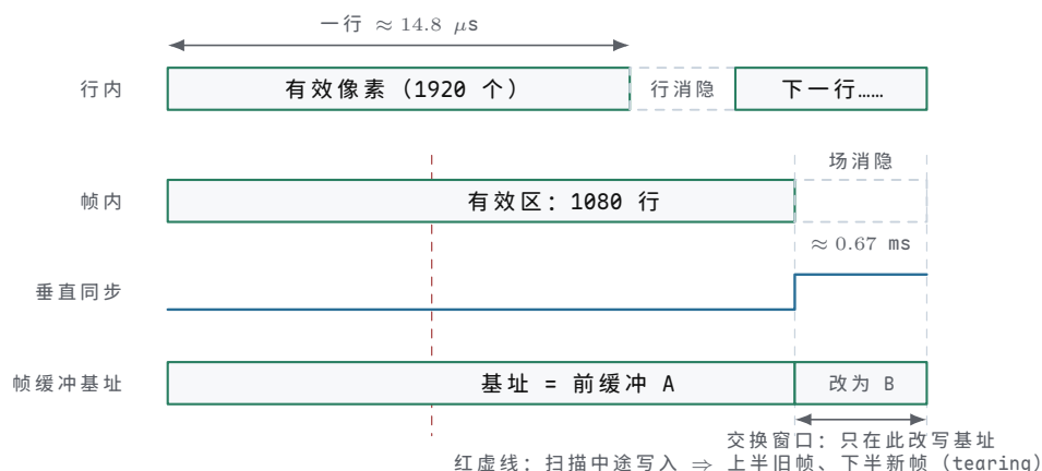
图示：显示扫描的两层时序（示意，不按比例）：行内先发有效像素再入行消隐，一行约 14.8 \mu\text{s} ；帧内扫完 1080 个有效行入场消隐，垂直同步脉冲随之拉高。双缓冲的交换—改写帧缓冲基址寄存器—只允许发生在场消隐窗口内；若在扫描中途改写（红虚线），屏幕上半是旧帧、下半是新帧，这就是 tearing。
