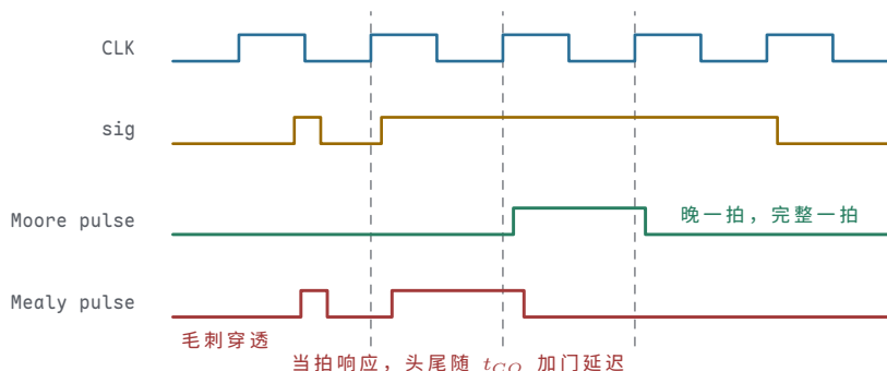
图示：同一 sig 下的两种输出：Mealy 在采到上升沿的当拍拉高，抢回一个周期，但 sig 上的窄毛刺原样穿透（左侧红色小脉冲），且脉冲头尾要等沿后 t_{CQ} 加一级门延迟，不如 Moore 整齐；Moore 晚一个周期进入 S_EDGE ，输出
