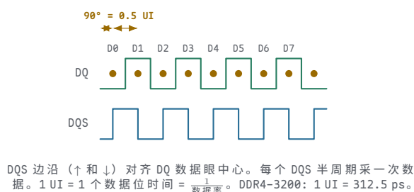
图示：DQS/DQ 对齐关系。DQS 相对 DQ 偏移 90^\circ (即四分之一 DQS 周期， 0.5\text{ UI} )，使 DQS 的上升沿和下降沿恰好落在 DQ 数据有效窗口的中心。
