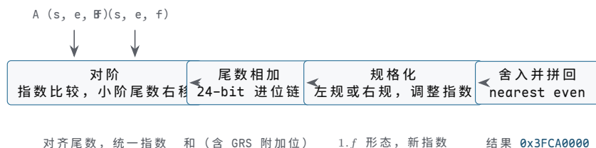
图 5-10 浮点加法四步的输入输出：对阶按指数差把小阶尾数右移，移出位进入 guard、round、sticky 附加位；尾数相加走普通整数进位链；规格化把结果移回 1.f 形态并同步加减指数；舍入按 round to nearest even 处理附加位后拼回 s/e/f 三段。四步次序固定，真实 FPU 把它们分到不同流水级。
