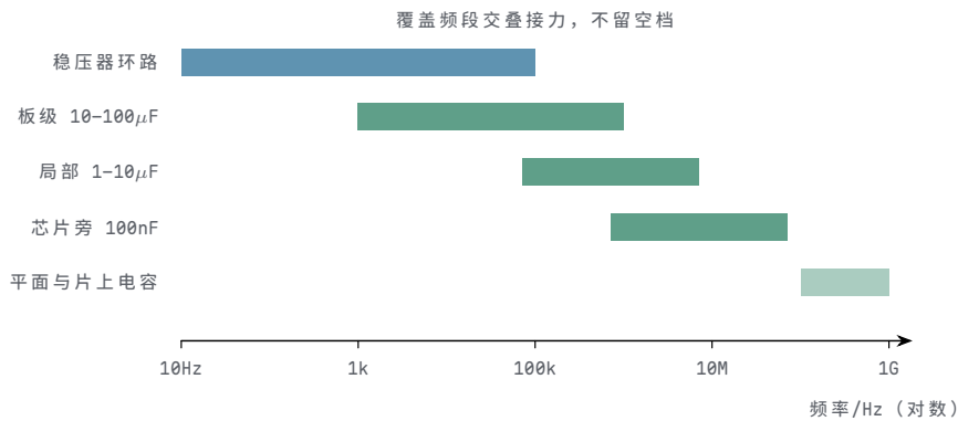
图示：去耦网络按时间尺度分层。储能自上而下逐层减小、响应逐层变快：每层只管自己来得及管的事件，耗尽之前由下一层补仓，最慢的部分留给稳压器环路。
