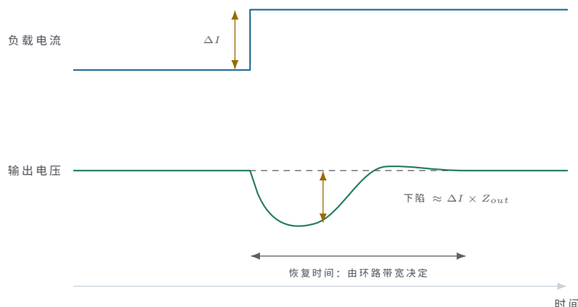
图示：负载电流阶跃下的 VRM 输出电压。最初的陡跌由输出电容的寄生电阻决定，环路来不及参与；随后的下滑与回升才是环路带宽的表演时间。带宽越高的环下陷越浅、恢复越快，但带宽受 LC 谐振与相位裕度限制，不能无限推高。
