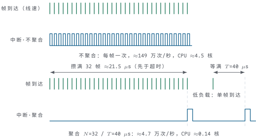
图示：中断聚合的时序对比。上方不聚合：每帧一次中断，1.49 Mpps 折合每秒约 149 万次中断进出，约 4.5 颗核的算力全花在保存与恢复现场上。下方聚合：攒满 32 帧（线速下约 21.5\ \mu\text{s} ，先于超时）或等满 T=40\ \mu\text{s} ——先到为准——才发一次中断，中断率降到约 4.7 万次/秒，CPU 开销约 0.14 核；代价是一帧平均多等约半个聚合窗口。
