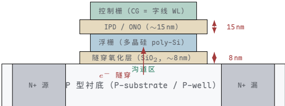
浮栅 NAND 单元截面（沿沟道方向）。N+ 源/漏之间是 P 型沟道；浮栅被隧穿氧化层（下）和 ONO 层间介质（上）完全包围，形成电荷势阱。
