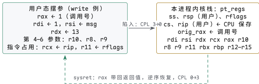
图示：系统调用的参数传递与现场保存（write(1, msg, 13) 例）。用户态按 ABI 摆好 rax 编号与 rdi/rsi/rdx 参数； syscall 指令把返回地址装进 rcx 、标志装进 r11 ——这正是第四个参数改用 r10 的原因——并把 rip 换成 LSTAR 入口。入口代码切到本进程内核栈，把用户态现场连同全部通用寄存器存成 pt_regs ，内核 C 代码看到的“寄存器”就是这张内存表； sysret 逆序恢复，返回值仍由 rax 带回，一进一出同一个寄存器。
