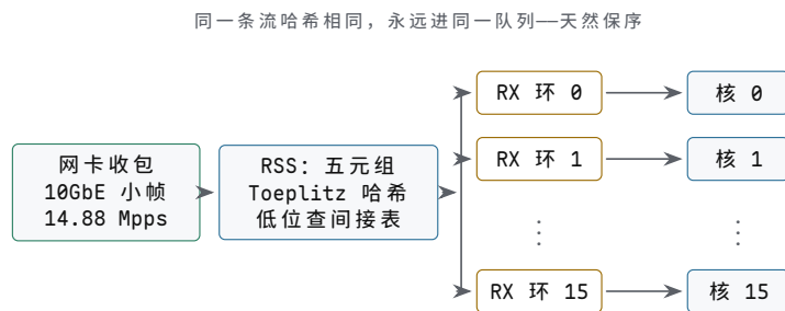
每对环绑一个 MSI-X 向量、绑一颗核；单核约 1.5 Mpps，16 颗核并行才接得住 14.88 Mpps
