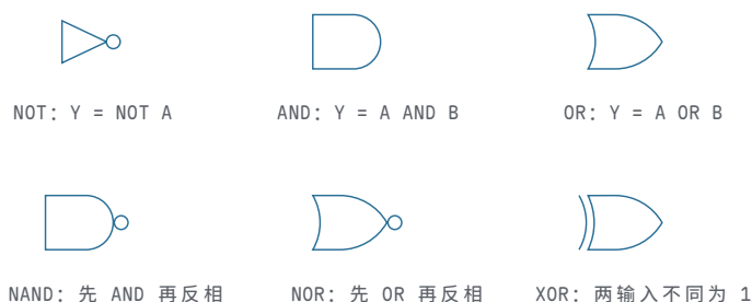
图 2-1 六个基本门的标准符号（美式画法）。注意输出端的小圆圈：它表示反相——NAND 就是 AND 加一个小圆圈，NOR 就是 OR 加一个小圆圈。这个小圆圈和晶体管开关模型里 PMOS 控制端的圆圈是同一个约定：有圈即取反。
