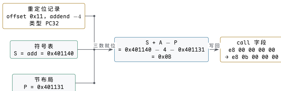
图示：重定位修补流水线（对应正文 main.o 调用 add 的演算）。链接器读出记录的位置、类型与加数，从符号表取 S 、从节布局取 P ，按类型公式代入：PC32 写入 S+A-P = 0x401140 - 4 - 0x401131 = 0x0B ；结果按小端排布写回字段， e8 00 00 00 00 变成 e8 0b 00 00 00 。RELA 格式下字段旧内容直接丢弃，整个修补就是一次减法加一次写字节。
