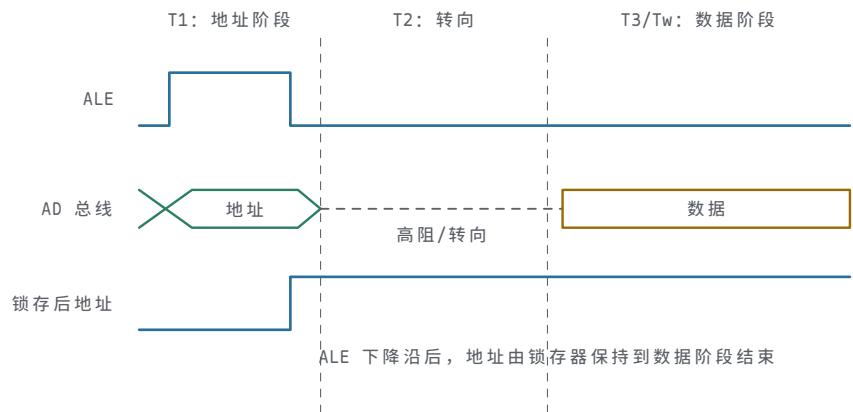
图示：8086 复用总线的一个读周期：T1 时 ALE 打开锁存窗口，地址随 AD 总线进入锁存器；ALE 落下后窗口关闭，AD 总线转向传数据，而锁存器把地址保持到 T3 采样完成。锁存器把一个总线相位的值变成后续相位仍然可用的状态。
