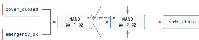
图 1.10 用两路 NAND 实现 AND。第二路 NAND 的两个输入接同一个反相信号，等价于把第 1 路输出再反相。图中分成两条回入线，是为了避免箭头穿过文字。
