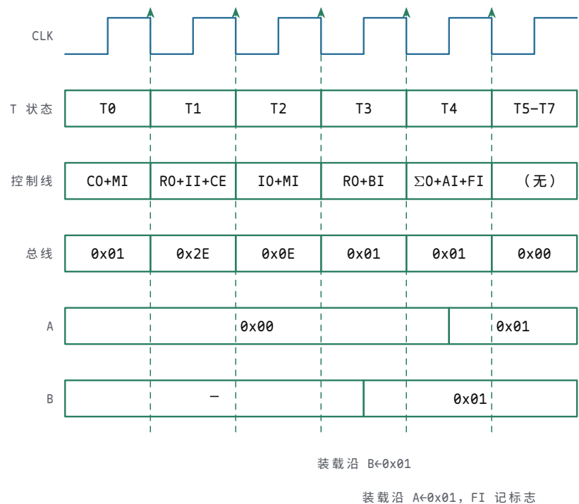
图示：程序一第二条指令 ADD 14 的 T0-T4 (第一圈: A=0x00, i=RAM[14]=0x01)。T0、T1 是公共取指：总线依次是 PC 的 0x01 和指令字节 0x2E; T2 总线是 IR 低 4 位 0x0E, 拍末 MAR←14; T3 总线是 RAM[14] 的 0x01, 拍末 B←0x01; T4 \Sigma 0 把 A+B=0x01 放上总线, 拍末 AI 收回 A、FI 锁存标志。参考虚线是 T 状态翻转的下降沿: B 在 T3 的装载沿 (拍内上升沿) 更新, A 在 T4 的装载沿更新, 控制字与总线值在装载沿前半拍已经稳定。
