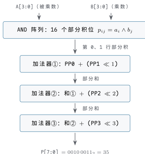
图示： 4 \times 4 阵列乘法器结构：16 个 AND 门一次生成全部部分积位，三行 4-bit 加法器逐行累加，每行按乘数位权重错开一位（ \ll 1 、 \ll 2 、 \ll 3 ）。 4 \times 4 需要 16 个 AND 门和约 12 个全加器； 0111 \times 0101 经三行累加得 0010\,0011_2 = 35 。
