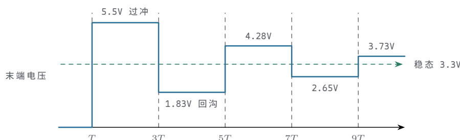
图示：3.3V、50Ω 走线、源阻 10Ω、末端开路时的末端电压逐拍演算。入射 2.75\text{V} 在 t = T 到达末端并全反射成 5.5\text{V} ，回波在源端被负反射后逐拍抵消，每往返一圈幅度乘 2/3 ，最终收敛到稳态 3.3V。
