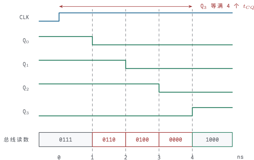
图示：4-bit 纹波计数器从 0111 计到 1000（每级 t_{CQ} = 1\text{ns} ）：CLK 沿后 1ns Q_0 先翻成 0，它的变化再触发 Q_1 ，逐级传递到 Q_3 已是沿后 4ns。底部总线行依次读出 0111、0110、0100、0000、1000——红色三格是计数序列中不存在的中间值，后级译码逻辑在这个窗口读数就会看到幻影。同步计数器所有位共享时钟，沿后一步整体更新，没有这些格子。
