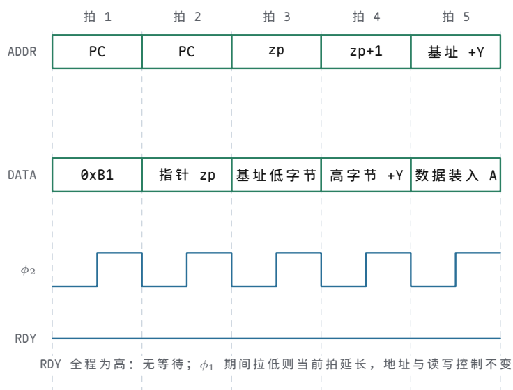
图示：LDA (zp),Y 的五拍总线时序：五拍全为读周期，每拍地址先送上总线，数据在 \phi_2 窗口内由存储器驱动，CPU 在 \phi_2 结束前采样。第 4 拍读基址高字节的同时，低字节与 Y 相加形成最终地址；RDY 全程为高，故没有任何等待拍。
