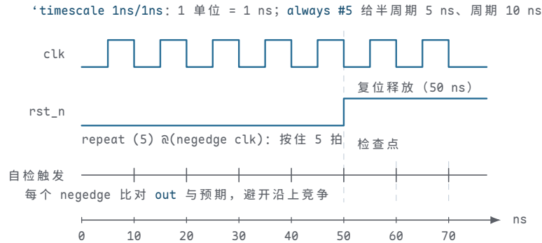
图示：仿真时间轴与三段代码的对应：‘timescale 1ns/1ns 把 1 个时间单位定为 1 ns，always #5 产生周期 10 ns 的时钟；复位拉低后经 repeat (5) @(negedge clk) 按住 5 拍，在第 5 个下降沿（50 ns）释放——刻意选在低电平期间，远离采样沿；自检块在每个下降沿比对 out 与预期，同样避开沿上的读写竞争。RTL 仿真里时间是离散的，这条轴上的每一格都是事件队列里的一个时刻。
