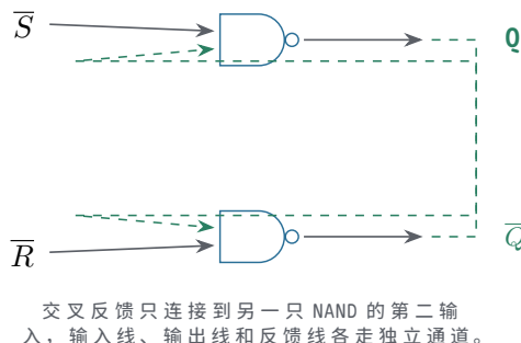
图示: 由两个交叉耦合的 NAND 门构成的 SR 锁存器。 \bar{S} 与 \bar{R} 低有效; 当两者都为高时, 反馈维持原状态。
