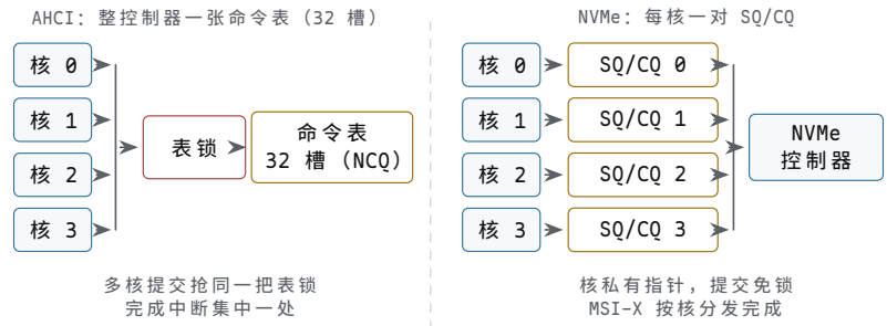
图示：AHCI 与 NVMe 的提交结构对照。AHCI 整台控制器只有一张 32 槽命令表（NCQ 深度 32）：所有核的提交抢同一把表锁，完成中断也集中在一处；SATA 的 600 MB/s、约十万 IOPS 下这张表不是瓶颈，PCIe SSD 把带宽抬高一个数量级、IOPS 抬高两个数量级之后，提交路径上的共享状态先成为瓶颈。NVMe 把表拆开：每核一对 SQ/CQ，尾指针核私有、提交免锁，完成由 MSI-X 按核分发—多队列是把那张唯一的表拆开之后的必然形态。
