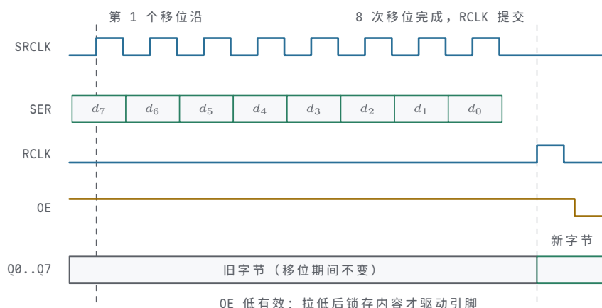
图示：74HC595 串并转换时序（括号内为部分手册别名：SER=DS、SRCLK=SHCP、RCLK=STCP）：SRCLK 的 8 个有效沿把 SER 上的 d_7 到 d_0 逐位移入内部移位寄存器，期间输出锁存器保持旧字节，外部引脚纹丝不动；8 次移位完成后给一个 RCLK 沿，整字节一次性提交到 Q0..Q7 ；OE 低有效，拉低之前引脚呈高阻。内部状态推进与外部可见提交分开，正是这颗芯片输出不抖的原因。
