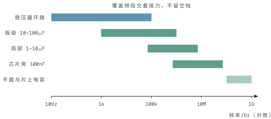
图示：各层电容在频率轴上的分工。稳压器环路管 100kHz 以下的慢变化；板级电解、局部 \mu F 级、芯片旁 100nF 按各自自谐振频率错开接力—10 \mu F 自谐振约 0.7MHz，100nF 约 7MHz；100MHz 以上分立电容无能为力，由电源-地平面对的平面电容与片上电容收尾。相邻层的覆盖频段交叠，合成阻抗曲线才不会在任何频段冒过目标线。
