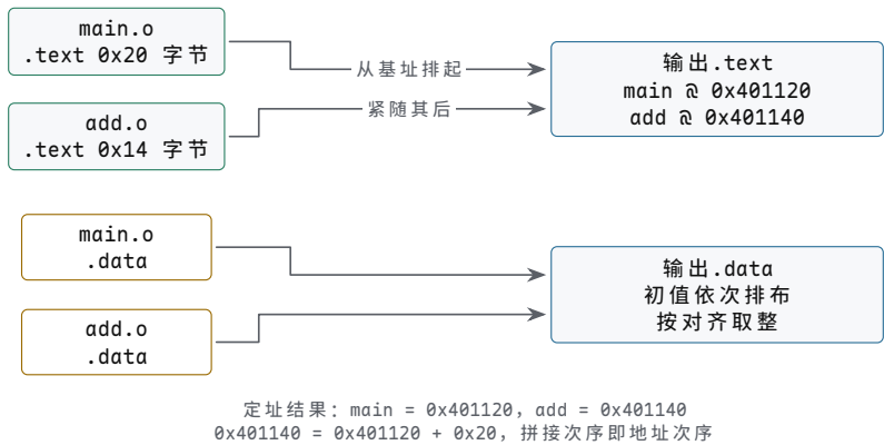
图示：静态链接的地址形成（对应正文 main.o 与 add.o 的最小例）。链接器把各输入文件的同类节依次拼接成输出的节： main.o 的 .text (0x20 字节) 铺在基址 0x401120 ， add.o 的 .text (0x14 字节) 紧随其后从 0x401140 开始；数据节同样处理。拼接完成，每个符号的值便从“节内偏移”换算成“节基址加偏移”的具体数—— main = 0x401120 ， add = 0x401140 ，重定位所需的 S 至此全部就位。
