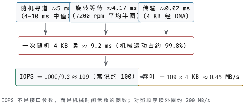
图示：随机 4 KB 读的 IOPS 换算链：随机寻道约 5 ms 加平均半圈的旋转等待约 4.17 ms，再加 4 KB 传输约 0.02 ms，合计约 9.2 ms；IOPS 是它的倒数，约 109，乘 4 KB 得吞吐约 0.45 MB/s——与顺序读外圈约 200 MB/s 差两个数量级。容量规划要从每盘约 100 IOPS 起步，而不是从标称带宽起步。
