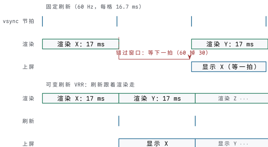
固定刷新: 上屏只能取节拍约数 (60/30/20); VRR: 帧率连续, 代价是帧间隔不均匀
