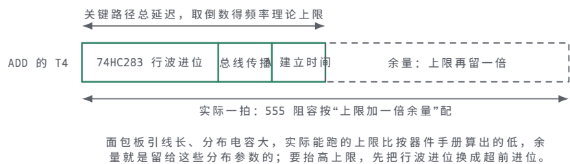
图示：整机性能预算：ADD 的 T4 是全机最长的一拍，关键路径由 74HC283 的行波进位 (8 位逐级传递)、总线传播和 A 寄存器建立时间三段串联而成，总延迟取倒数就是时钟频率的理论上限。实际配置再留一倍余量——分段条右半的虚线部分，555 的阻容按这个加了余量的周期来配。
