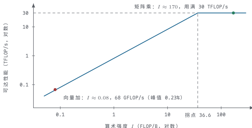
图示: 双对数坐标下的 roofline: 斜段是带宽屋顶(可达性能 = 带宽 × 算术强度), 平段是算力屋顶 30 TFLOP/s, 拐点 I^* = 30000/820 \approx 36.6 FLOP/B。向量加的强度只有约 0.08 FLOP/B, 被带宽屋顶压在 68 GFLOP/s—峰值的 0.23%; 矩阵乘约 170 FLOP/B, 远在拐点右侧, 峰值真正用满。横轴每往左一格, 同样的算力折扣再重一倍。
