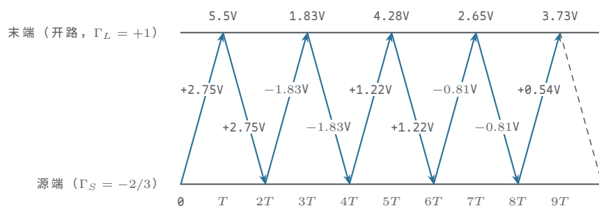
图示：弹跳图：横轴时间、纵轴位置，斜线是行波在源端与末端之间的来回，每跨一次耗时 T 。入射 +2.75\text{V} 在 t = T 到达开路末端， \Gamma_L = +1 全反射，末端跳到 5.5\text{V} ；回波在源端按 \Gamma_S = -2/3 反号弹回，每往返一圈幅度乘 2/3 。上轨标出的各时刻末端电压 5.5、1.83、4.28、2.65、3.73V 与上表逐项一致，逐拍收敛到稳态 3.3V。
