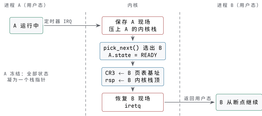
图示：上下文切换泳道（对应正文 trace）。定时器中断在指令边界把 CPU 从 A 带进内核：A 的现场压上它自己的内核栈，调度器选出 B 后写入 B 的页表基址（CR3）、把栈指针切到 B 的内核栈，再弹出 B 的寄存器并 iretq ——返回落进 B 的用户态，B 只得上次陷入返回得特别久。被切走的 A，全部状态归结为进程控制块里的一个栈指针，等下次被选中时原路恢复。
