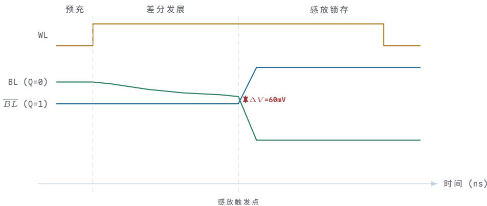
读操作时序：WL 打开后 BL 缓慢放电（Q=0 侧）， \overline{BL} 保持高（Q=1 侧）。差分电压超过感放的最小可辨阈值（灵敏度下限，约 50-80mV，远大于失调电压）后，正反反馈在 0.3ns 内放大到全摆幅。
