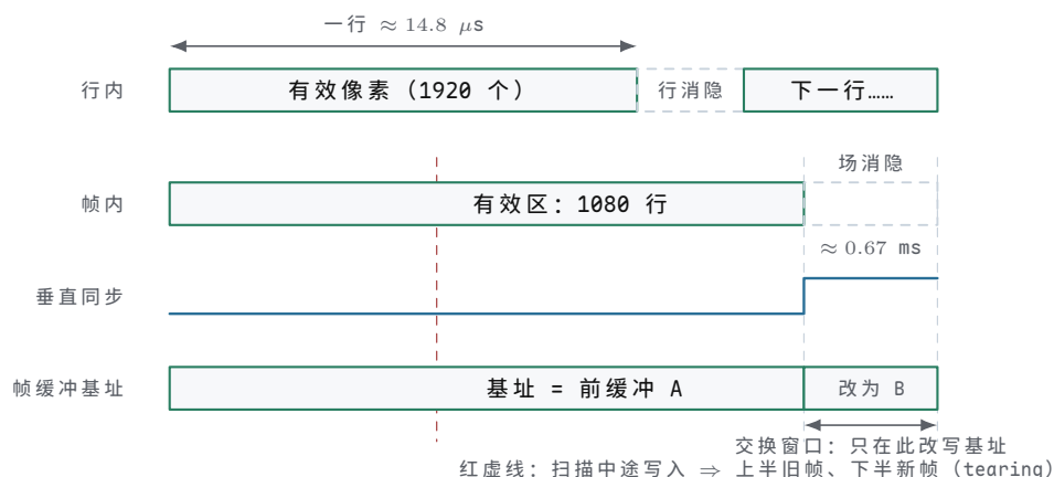
图示：显示扫描的两层时序（示意，不按比例）：行内先发有效像素再入行消隐，一行约 14.8\text{ }\mu\text{s} ；帧内扫完 1080 个有效行进入场消隐，垂直同步脉冲随之拉高。双缓冲的交换——改写帧缓冲基址寄存器——只允许发生在场消隐窗口内；若在扫描中途改写（红虚线），屏幕上半是旧帧、下半是新帧，这就是 tearing。
