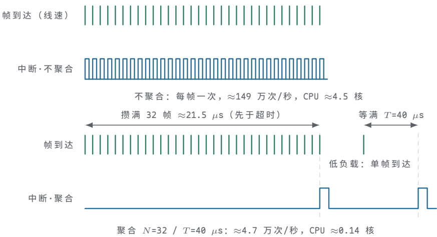
图示：中断聚合的时序对比。上方不聚合：每帧一次中断，1.49 Mpps 折合每秒约 149 万次中断进出，约 4.5 颗核的算力全花在保存与恢复现场上。下方聚合：攒满 32 帧（线速下约 21.5 μs，先于超时）或等满 T=40 μs——先到为准——才发一次中断，中断率降到约 4.7 万次/秒，CPU 开销约 0.14 核；代价是一帧平均多等约半个聚合窗口。
