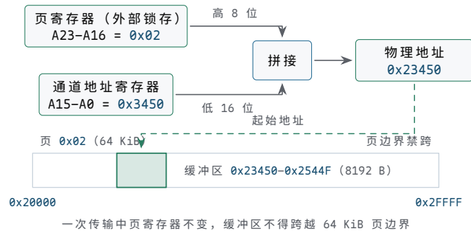
图示：8237 的 24 位地址拼接：外部页寄存器锁存 A23-A16，通道地址寄存器提供 A15-A0。示例页号 0x02、页内偏移 0x3450 合成物理地址 0x23450；8192 字节传到 0x2544F 为止，仍在页 0x02 (0x20000-0x2FFFF) 之内。一次传输中页寄存器保持不变，跨 64 KiB 页边界的缓冲区必须拆成两次传输。
