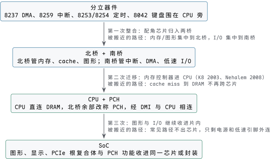
图示：芯片组演进链：每一次迁移搬近的都是某条具体路径——先是配角芯片归入南北两桥，再是内存控制器进 CPU，让 cache miss 到 DRAM 不再跨芯片（收益最大的一次，因为取指和读数是整机里最频繁的路径），最后图形、PCIe 根复合体和 PCH 功能收进 SoC。中断和 DMA 这类本来就慢的路径一直留在南侧。
