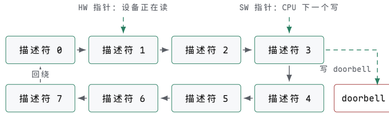
图示：描述符环。设备按 HW 指针顺序消费，CPU 按 SW 指针顺序生产，描述符 7 之后回到 0；CPU 更新 SW 后写一次 doorbell 提示设备。完成与否以设备写回描述符状态位为准，doorbell 只是“有新描述符”的提示。
