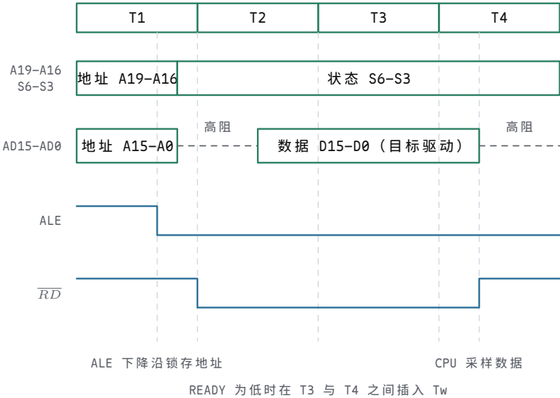
图示：8086 存储器读周期波形。T1 输出地址并拉高 ALE，地址锁存器在 ALE 下降沿保存地址；T2 复用脚转入数据方向，RD 拉低；T3 由目标芯片驱动数据线，READY 不满足则在 T3 与 T4 之间插入 Tw；T4 CPU 采样数据，控制信号撤销。同一组 AD 引脚在一个周期内先后是地址、高阻、数据—复用总线的每一拍都有唯一驱动者。
