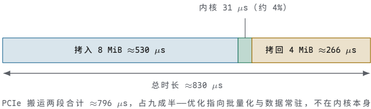
图示：一次内核启动的耗时构成（ N = 2^{20} 向量加，PCIe 3.0 x16，按比例）：拷入 8 MiB 约 530 \mu s，内核执行约 31 \mu s，拷回 4 MiB 约 266 \mu s，总时长约 830 \mu s。两次 PCIe 搬运占九成半，内核只占约 4%——算术强度约 0.08 FLOP/B 的负载，时间几乎全花在搬运上；工程上要么批量化、让数据常驻显存把这笔固定开销摊薄，要么干脆留在 CPU 上。
