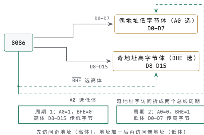
图 8-2 8086 的字节存储体：偶地址字节在低体，接 D0-D7，由 A0=0 选中；奇地址字节在高体，接 D8-D15，由 \overline{BHE} =0 选中。偶地址字访问两体同时选中，一个总线周期完成；奇地址字访问拆成两个周期：先 A0=1、 \overline{BHE} =0 经高体传字的低字节，地址加一后 A0=0、 \overline{BHE} =1 经低体传字的高字节。
