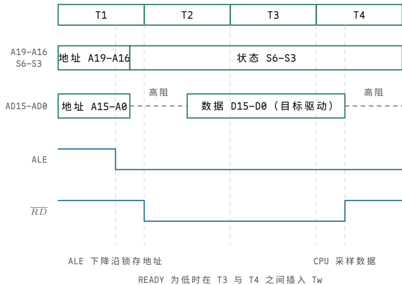
图 8-1 8086 存储器读周期波形。T1 输出地址并拉高 ALE，地址锁存在 ALE 下降沿保存地址；T2 复用脚转入数据方向， \overline{RD} 拉低；T3 由目标芯片驱动数据线，READY 不满足则在 T3 与 T4 之间插入 Tw；T4 CPU 采样数据，控制信号撤销。同一组 AD 引脚在一个周期内先后是地址、高阻、数据—复用总线的每一拍都有唯一驱动者。
