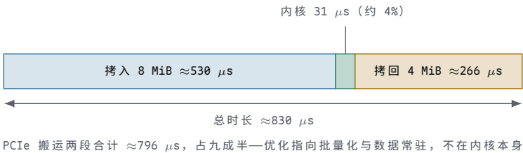
图示：一次内核启动的耗时构成（ N = 2^{20} 向量加，PCIe 3.0 x16，按比例）：拷入 8 MiB 约 530 \mu s，内核执行约 31 \mu s，拷回 4 MiB 约 266 \mu s，总时长约 830 \mu s。两次 PCIe 搬运占九成半，内核只占约 4%—算术强度约 0.08 FLOP/B 的负载，时间几乎全花在搬运上；工程上要么批量化、让数据常驻显存把这笔固定开销摊薄，要么干脆留在 CPU 上。
