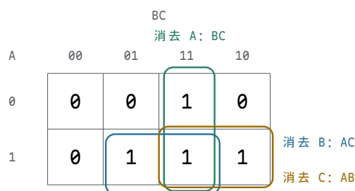
图示：三变量卡诺图（注意列头顺序 00、01、11、10 是 Gray 码：相邻两列永远只差一个 bit，这样“相邻”才有消元意义）。三个圈各合并两个相邻的 1：每个圈里那个“两种取值都出现”的输入被消去，得到 Y = AB \text{ OR } AC \text{ OR } BC ——与后文三传感器判断器用最小项硬推出的结果一致，但快得多。
