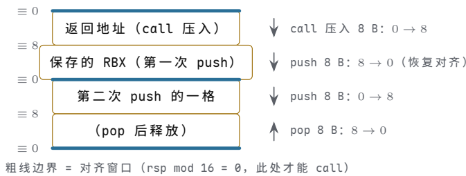
图示：栈按 8 字节为一格，高地址在上。每次 push 或 call 压入一格，rsp mod 16 的余数就翻转一次；pop 弹出一格，余数再翻转回来。call 要求执行瞬间余数为 0——图中粗线标出的对齐窗口；call 压入返回地址后，被调用函数入口处的余数变为 8，序言用奇数次 push（或一条 sub rsp, 8）把余数调回 0，下游的 call 才落在对齐窗口上。
