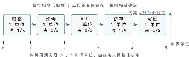
最坏指令（加载）：五段组合路径在一拍内相继稳定
