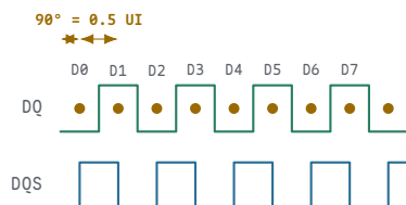
DQS 边沿 (↑ 和 ↓) 对齐 DQ 数据眼中心。每个 DQS 半周期采一次数据。1 UI = 1 个数据位时间 = \frac{1}{\text{数据率}} 。DDR4-3200: 1 UI = 312.5 ps。
