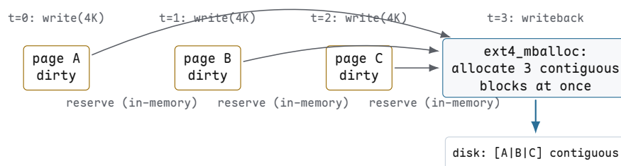
图示：延迟分配时间线。三次 write() 调用仅在内存中预留空间。写回时， ext4_mballoc 一次性为所有脏页分配连续物理块，实现最优布局。
