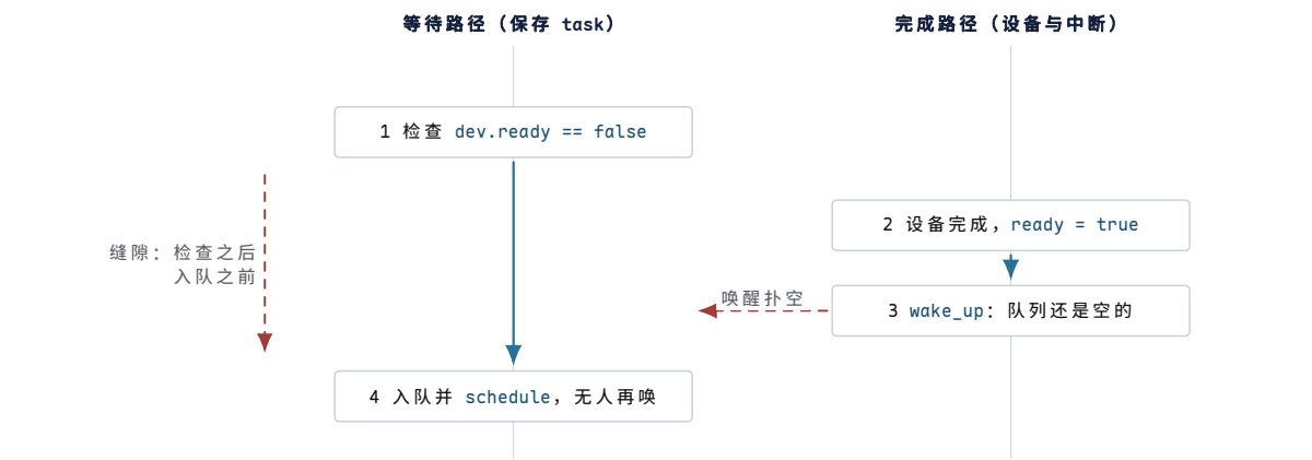
图示：两条路径各自都“做了正确的事”，错误出在缝隙里：完成事件恰好落在等待者检查条件之后、登记入队之前。把检查和入队放进同一个受保护区间，缝隙才被封死。
