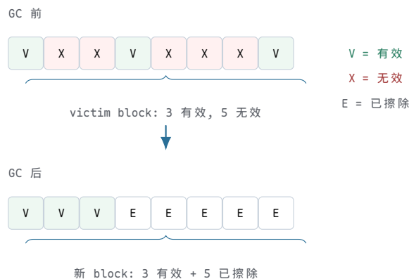
FTL 垃圾回收过程
