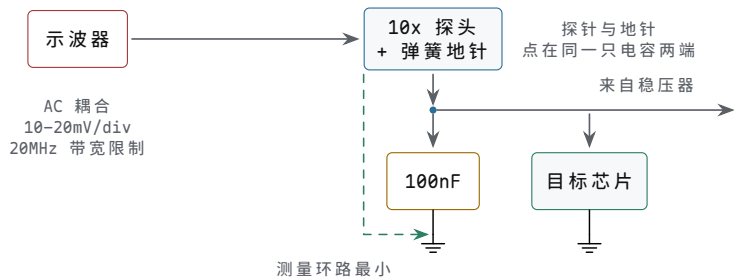
图示：纹波测量的标准接法。示波器切 AC 耦合挡住直流分量，用 10-20mV/div 的档位把纹波展开；10x 探头配弹簧地针，探针与地针直接点在该目标芯片电源脚旁那只去耦电容的两端——测的是负载端真实看到的电源，探头围出的测量环路也最小；示波器若有 20MHz 带宽限制就打开，挡住与电源无关的高频拾取。
