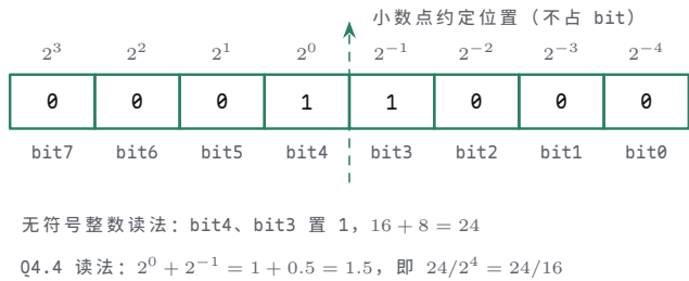
图示：同一个 8-bit 模式 00011000 在 Q4.4 约定下的位权解读。电路里的 8 个 bit 不变，约定把小数点固定在 bit 4 与 bit 3 之间：高 4 位权重 2^3 到 2^0 ，低 4 位权重 2^{-1} 到 2^{-4} 。置 1 的是 bit4 与 bit3，按整数读为 16 + 8 = 24 ，按 Q4.4 读为 1 + 0.5 = 1.5 ——两种读法相差的正是缩放因子 2^4 ，即 24/16 = 1.5 。
