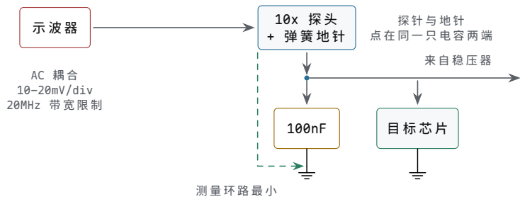
图示：纹波测量的标准接法。示波器切 AC 耦合挡住直流分量，用 10–20mV/div 的档位把纹波展开；10× 探头配弹簧地针，探针与地针直接点在被测芯片电源脚旁那只去耦电容的两端——测的是负载端真实看到的电源，探头围出的测量环路也最小；示波器若有 20MHz 带宽限制就打开，挡住与电源无关的高频拾取。
