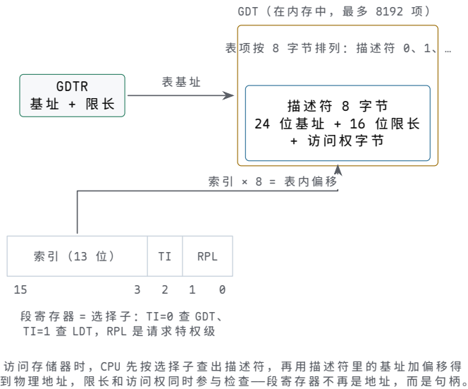
图示：80286 保护模式的选择子与描述符。段寄存器的高 13 位是描述符表内索引，每项 8 字节，索引乘 8 得表内偏移；TI 位选 GDT 还是 LDT；低 2 位是请求特权级。GDTR 保存 GDT 的基址和限长，描述符装着 24 位段基址、16 位限长和访问权字节——查表得到基址再加偏移，才是最终的物理地址。
