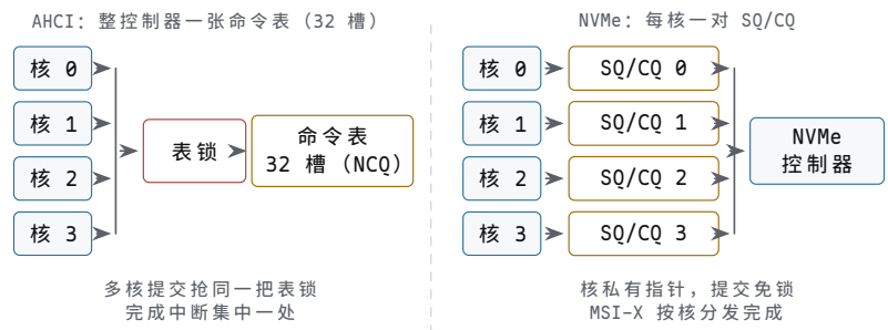
图示：AHCI 与 NVMe 的提交结构对照。AHCI 整台控制器只有一张 32 槽命令表 (NCQ 深度 32)：所有核的提交抢同一把表锁，完成中断也集中在一处；SATA 的 600 MB/s、约十万 IOPS 下这张表不是瓶颈，PCIe SSD 把带宽抬高一个数量级、IOPS 抬高两个数量级之后，提交路径上的共享状态先成为瓶颈。NVMe 把表拆开：每核一对 SQ/CQ，尾指针核私有、提交免锁，完成由 MSI-X 按核分发—多队列是把那张唯一的表拆开之后的必然形态。
