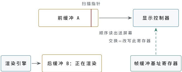
交换只在场消隐那 0.67 ms 内执行：一次寄存器写，零拷贝，A、B 角色互换
