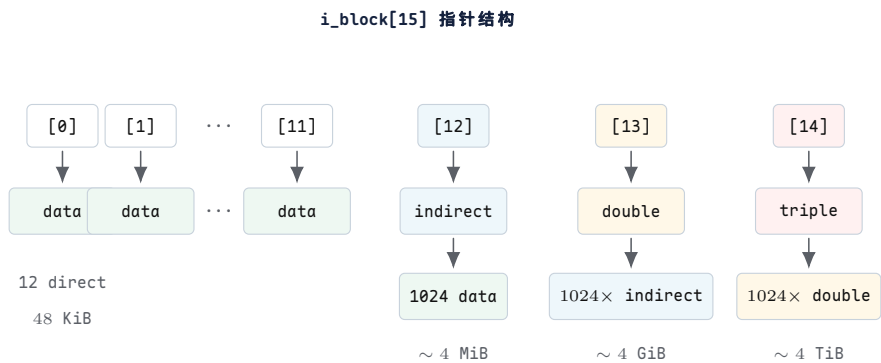
图示：蓝色 = 单重间接，琥珀色 = 双重间接，红色 = 三重间接，绿色 = 数据块。每个间接块包含 1024 个 4 字节指针（4096 / 4 = 1024）。颜色越深表示间接层级越多、寻址时需要的磁盘读次数越多。
