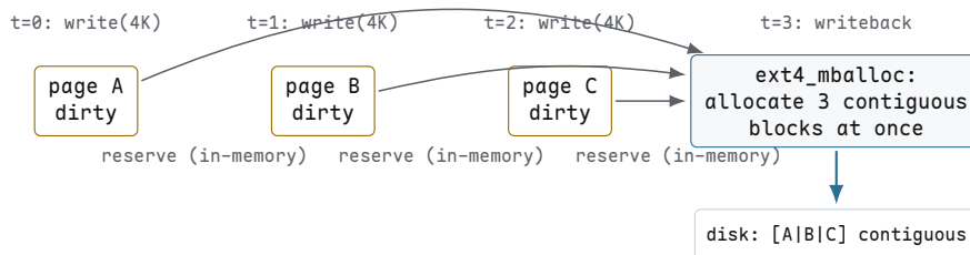
图示：延迟分配时间线。三次 write() 调用仅在内存中预留空间。写回时， ext4_mballoc 一次性为所有脏页分配连续物理块，实现最优布局。
