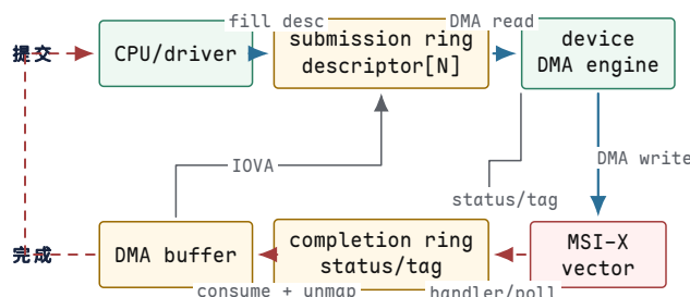
图示：队列型设备的通用结构：descriptor 在普通 RAM，doorbell 在 MMIO，数据通过 DMA，完成通过 completion ring 和 MSI-X 返回。
