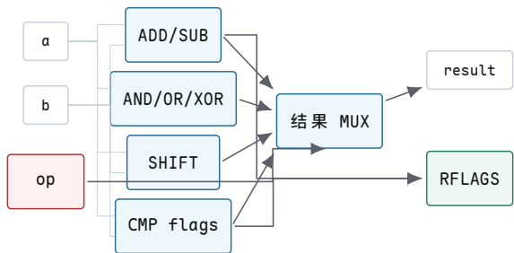
图示：ALU 由多种组合功能和结果选择器组成。控制信号选择输出，标志路径影响后续条件分支和异常返回。
