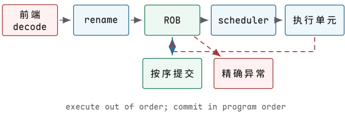
图示：乱序 CPU 的教学结构。rename 和 scheduler 提高并行度，ROB 保证 precise exception 和按序提交。
