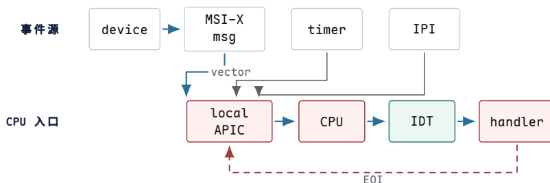
图示：中断投递链。设备事件先变成 vector，再由 CPU 查 IDT 进入入口；handler 完成后还要满足设备确认和 APIC EOI。
