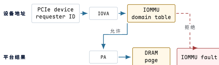
图示：IOMMU 把设备发出的 IOVA 翻译成物理地址，并按设备 domain 检查权限。没有映射或方向错误会形成 IOMMU fault。
