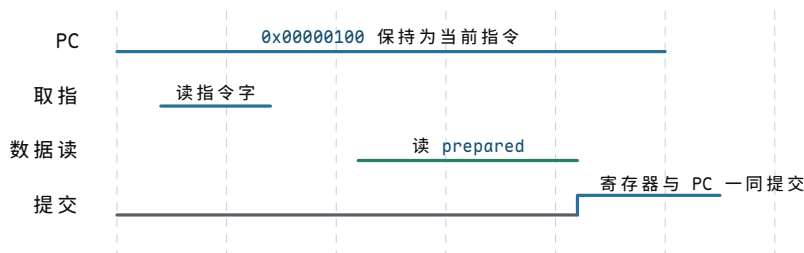
图示：PC 在数据读取等待期间仍指向产生该读取的指令。这使失败位置具有唯一含义。
