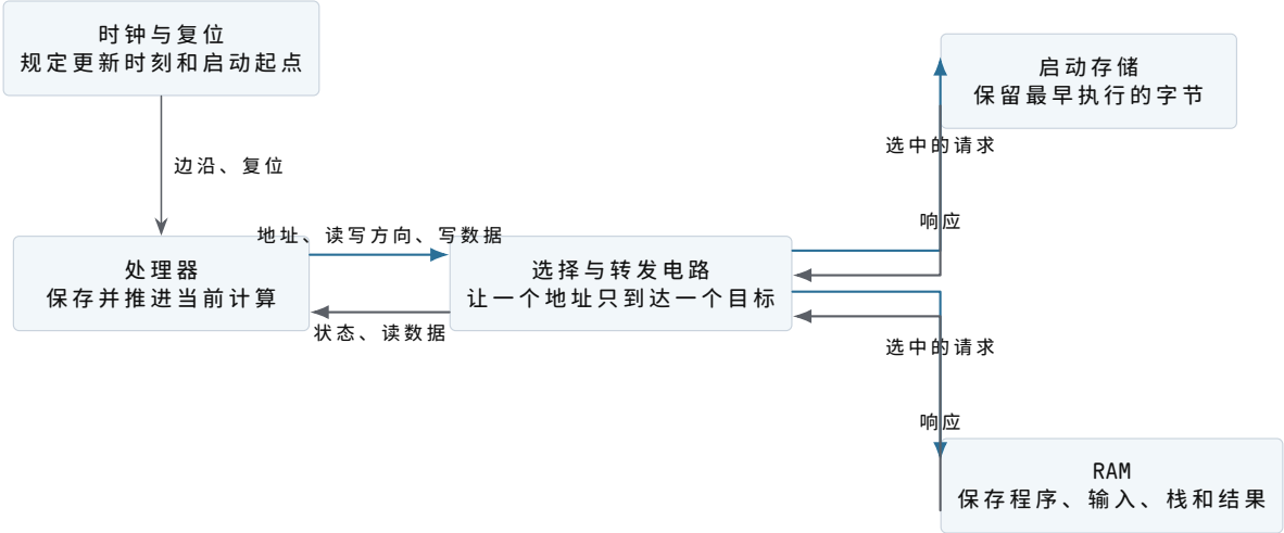
图示：图中只有当前真实存在的硬件。调试工具在复位期间预置 RAM，运行开始后退出；图中没有操作系统、调度器、系统调用或可编程计时器。
