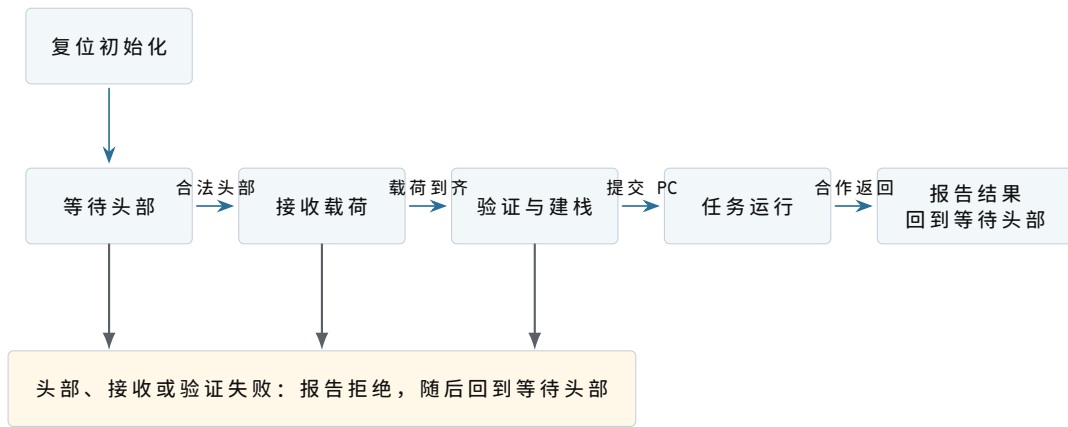
图示：上排是一次成功传输从左到右的状态变化，下排统一表示任务运行以前的拒绝路径。进入任务后，唯一正常出边仍是任务主动返回；当前机器没有从运行状态强制回到固件的事件。
