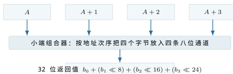
图示：字节顺序是处理器与存储接口之间的解释规则。RAM 单元只保存八个位，并不保存“最低有效字节”这个语义标签。
