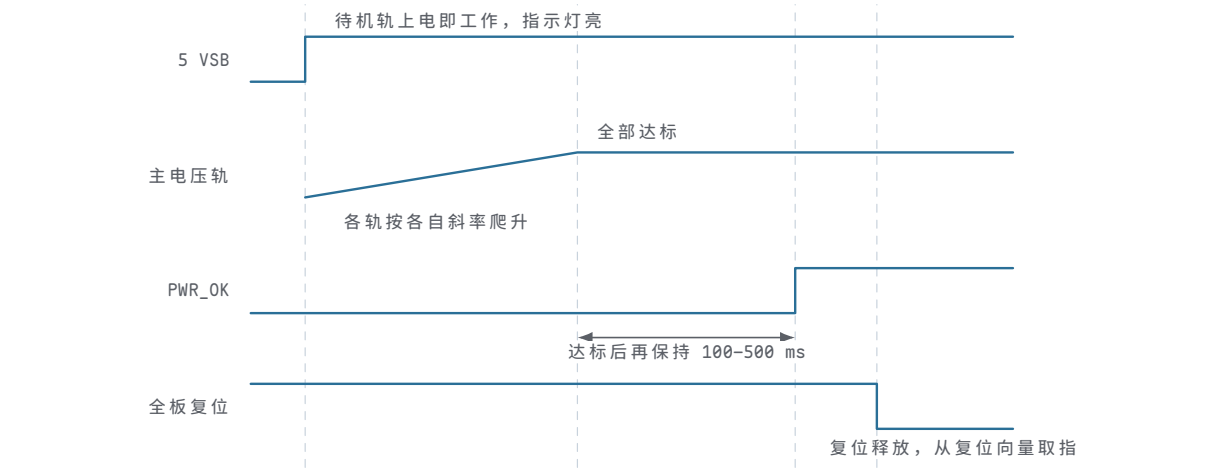
图示：主板电源时序：待机轨 5 VSB 上电即工作，主电压轨按各自斜率爬升，全部达标之后 PWR_OK 再保持 100~500 ms 才有效，复位电路以 PWR_OK 为释放条件、按时钟节拍释放复位树。指示灯亮只说明待机轨在工作，它与主电压轨稳定相差几十到几百毫秒——这就是“插电能亮”不等于“电压稳定”的时序根源。
