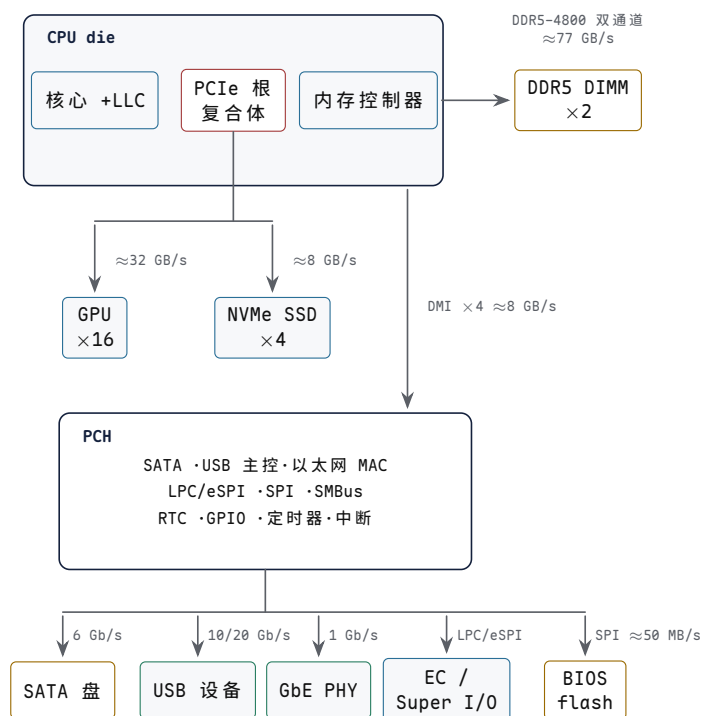
图示：现代 PC 平台拓扑与带宽量级（单向）。CPU die 内的内存控制器与 PCIe 根复合体接管最快的路径：DRAM 直连内存控制器，GPU 与 NVMe SSD 挂在根复合体上；PCH 经 DMI 汇聚全部低速 I/O。注意图上每一处带宽差距都在 10 倍以上——DRAM 约 77 GB/s，DMI 约 8 GB/s，SATA 约 600 MB/s，LPC 与 SPI 只有数十 MB/s——这个落差正是“快慢分桥”的原因。软件侧的直接对应： lspci -tv 输出的顶层设备 host bridge 与 ISA bridge，就是 CPU 内根复合体与 PCH 在 PCI 模型中的投影。
