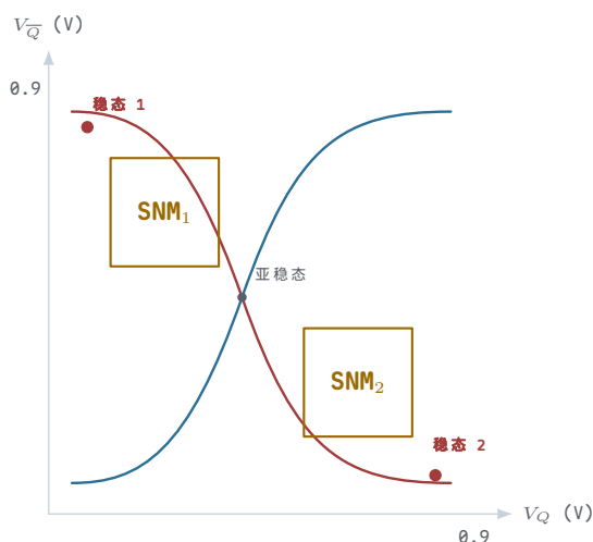
蝶形图：红色曲线为反相器 1 的 VTC，蓝色曲线为反相器 2 的镜像 VTC。两个“眼”中的最大内切正方形边长 = SNM。SNM = \min(SNM_1, SNM_2) 。工艺波动使两个眼不对称，较小者决定单元裕量。
