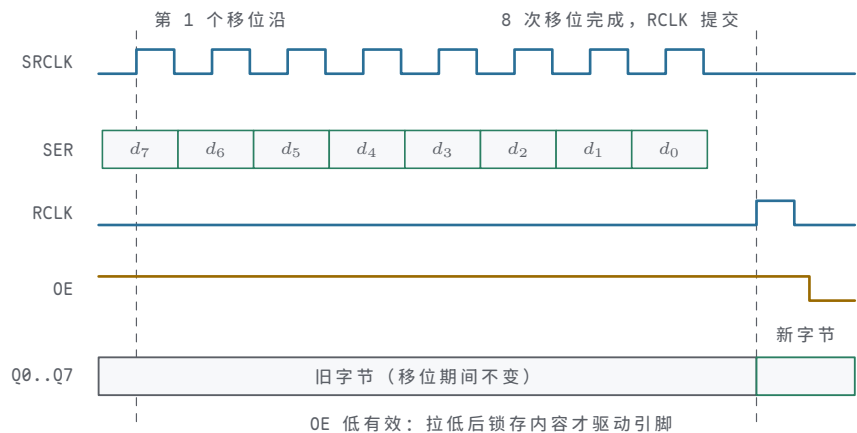
图示：74HC595 串并转换时序（括号内为部分手册别名：SER=DS、SRCLK=SHCP、RCLK=STCP）：SRCLK 的 8 个有效沿把 SER 上的 d_7 到 d_0 逐位移入内部移位寄存器，期间输出锁存器保持旧字节，外部引脚纹丝不动；8 次移位完成后给一个 RCLK 沿，整字节一次性提交到 Q0..Q7 ；OE 低有效，拉低之前引脚呈高阻。内部状态推进与外部可见提交分开，正是这颗芯片输出不抖的原因。
