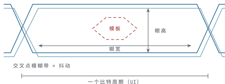
图 20-1 眼图的形成与读法：把数据波形按一个 UI 切段叠加，所有跳变轨迹交织出中央开口。眼高对应判决时刻的噪声裕量，眼宽对应采样点的时序裕量，交叉点的横向模糊带是抖动的直接读数；红色六边形是规范模板，任何轨迹都不得进入。
