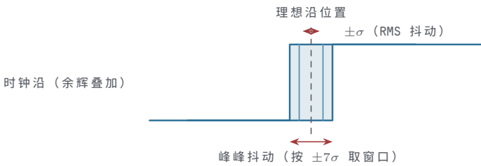
图示：抖动的直接图像：示波器余辉模式下，同一个时钟沿在理想位置两侧涂抹成一条带。带的散布宽度对应 RMS 抖动 \sigma ，时序预算按 \pm 7\sigma 的峰峰窗口扣除。
