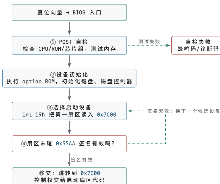
图示：BIOS 启动的四阶段流程：POST 失败时以蜂鸣码或诊断口代码报告，不进入后续阶段；选设备阶段按约定的启动顺序逐个尝试，签名无效就回到下一个候选设备；只有签名有效的扇区才能得到 CPU 控制权。
