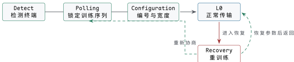
图示: PCIe 链路训练的主路径。链路只有进入 L0 后才能承载普通 TLP; Recovery 可以回到 L0, 也可以重新协商。设备“枚举不到”时, 首先要区分物理链路尚未进入 L0, 还是链路正常但配置事务失败。
