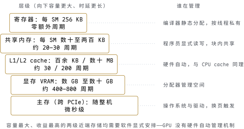
图示：GPU 存储层级与各级管理者。寄存器与共享内存这两级近端存储由编译器与程序员显式安排：寄存器按线程静态瓜分，多用一个变量就可能挤掉一整组驻留线程；共享内存由程序员写代码搬运与复用。L1/L2 仍由硬件自动管理，再往外是显存与跨 PCIe 的主存。与 CPU 全由硬件 cache 自动管理不同，GPU 将近端两级交由程序员显式管理——安排合理时效率更高，安排不当时也没有自动补偿机制。
