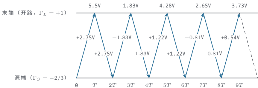
图示：弹跳图：横轴时间、纵轴位置，斜线是行波在源端与末端之间的来回，每跨一次耗时 T 。入射 +2.75\text{V} 在 t = T 到达开路末端， \Gamma_L = +1 全反射，末端跳到 5.5V；回波在源端按 \Gamma_S = -2/3 反号弹回，每往返一圈幅度乘 2/3 。上轨标出的各时刻末端电压 5.5、1.83、4.28、2.65、3.73V 与上表逐项一致，逐拍收敛到稳态 3.3V。
