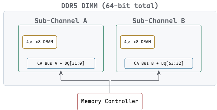
两个子通道完全独立：可以同时给 A 发 ACTIVATE、给 B 发 READ。每个子通道 32-bit DQ，BL16 仍输出 64 字节（一条 cache line）。
