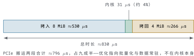
图示：一次内核启动的耗时构成（ N = 2^{20} 向量加，PCIe 3.0 x16，按比例）：拷入 8 MiB 约 530 \mu s，内核执行约 31 \mu s，拷回 4 MiB 约 266 \mu s，总时长约 830 \mu s。两次 PCIe 搬运占九成半，内核只占约 4%—算术强度约 0.08 FLOP/B 的负载，时间几乎全花在搬运上；工程上要么批量化、让数据常驻显存把这笔固定开销摊薄，要么干脆留在 CPU 上。
