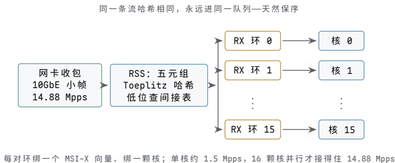
图示：RSS 接收分流：网卡对每帧的五元组算 Toeplitz 哈希，取低位查间接表，把帧定向到对应 RX 环；每对环绑一个 MSI-X 中断向量、绑一颗核，各核独立处理自己环上的帧，提交路径无锁。同一条流哈希相同、永远进同一队列，保序由哈希天然保证；并行度由队列对数决定—10 GbE 小帧 14.88 Mpps 对单核约 1.5 Mpps，16 队列绑 16 核才接得住。
