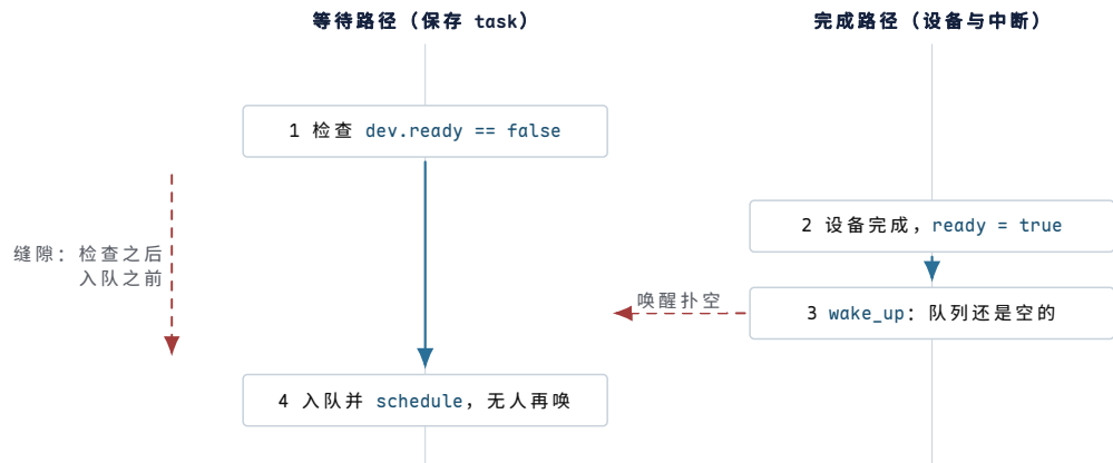
图示：两条路径各自都“做了正确的事”，错误出在缝隙里：完成事件恰好落在等待者检查条件之后、登记入队之前。把检查和入队放进同一个受保护区间，缝隙才被封死。
