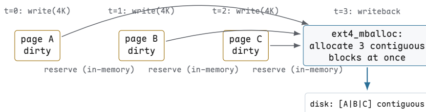
图示：延迟分配时间线。三次 write() 调用仅在内存中预留空间。写回时， ext4_mballo 一次性为所有脏页分配连续物理块，实现最优布局。
