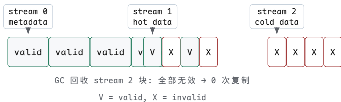
图示：NVMe 多流写入。不同生命周期的数据分配到不同流，SSD 内部将流映射到不同的擦除块组。当 GC 回收 stream 2 的块时，所有页已无效——零次有效页复制，写放大 = 1.0。
