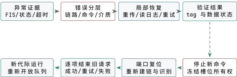
图示：错误恢复先尝试与失败层匹配的局部动作；只有错误持续或端口状态不再可信时，才冻结队列并复位端口。复位后仍要逐项处理旧 tag，再建立新代际并开放请求，不能把“链路重新起来”直接等同于所有旧命令都失败或都成功。
