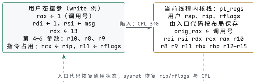
图示：系统调用的参数传递与现场保存（ write(1, msg, 13) 例）。用户态按 ABI 摆好 rax 编号与 rdi/rsi/rdx 参数； syscall 指令把返回地址装进 rcx 、标志装进 r11 ——这正是第四个参数改用 r10 的原因——并把 rip 换成 LSTAR 入口；它本身不保存用户 rsp ，也不自动切换栈。入口代码随后切到当前线程的内核栈，把用户态现场连同全部通用寄存器存成 pt_regs ，内核 C 代码看到的“寄存器”就是这张内存表；最后由 sysret 恢复 rip/rflags 与用户特权级，返回值仍由 rax 带回，一进一出同一个寄存器。
