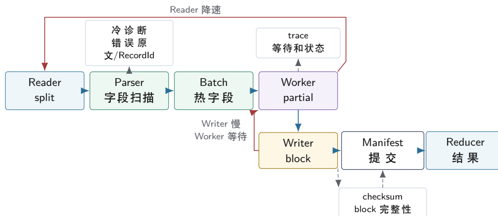
图示：端到端管线要同时看热路径、冷诊断、提交证据和背压方向；这样每个箭头都能连接到后续章节的实验。
