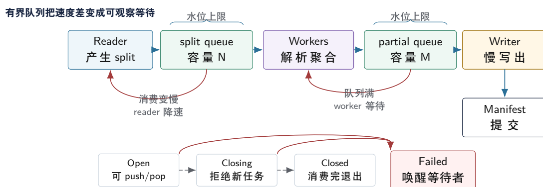
图示：背压不是把系统简单变慢，而是让队列长度、等待点、关闭路径和失败传播都进入可检查状态。
